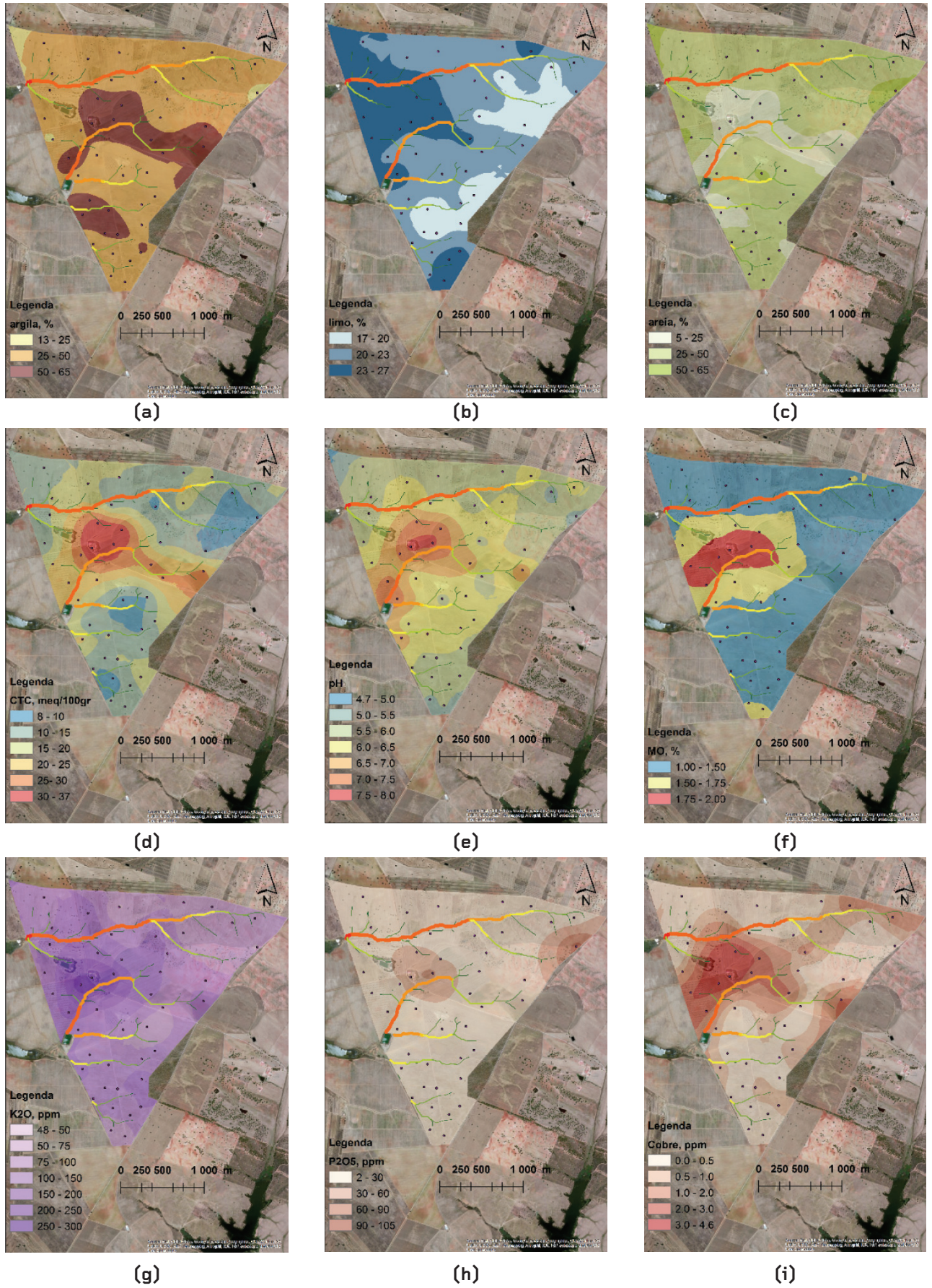
Figura 9. Variação espacial de propriedades do solo na “Herdeade de Linhares”: a) argila; b) limo; c) areia; d) capacidade de troca catiônica; e) pH; f) matéria orgânica; g) potássio; h) fósforo; i) cobre
