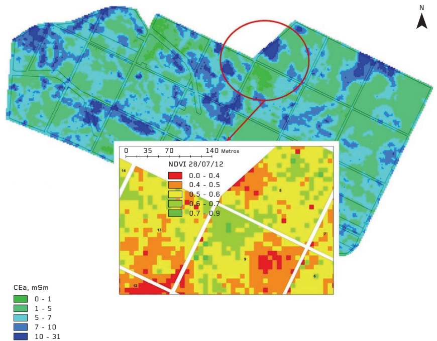
Figura 6. Pormenor da relação entre a CEa do solo e o vigor da vegetação (NDVI) na vinha do “Casito”
