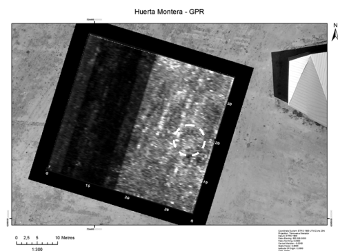
Figura 4 – Radargrama à profundidade temporal de 15 ns colocado e georreferenciado sobre a fotografia aérea do local de estudo (Radargram at temporal depth of 15 ns, placed and georeferenced over the aerial photograph of the study site).
