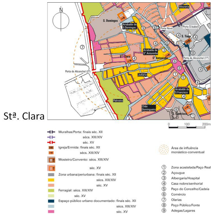
Fig. 3. Mosteiro de Santa Clara. Sobre planta do séc. XIX, evolução urbana da envolvente (reconstituição).
