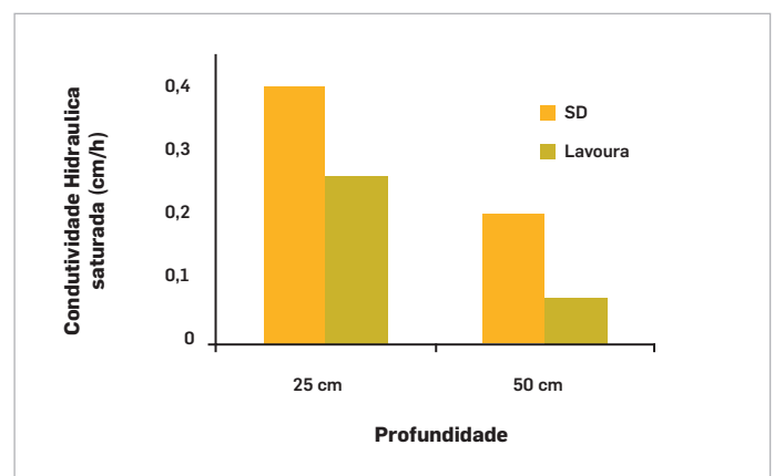
Figura 7 - Efeito do sistema de mobilização do solo na condutividade saturada de um Solo de Barro Preto, ao fim de seis anos de ensaio.
