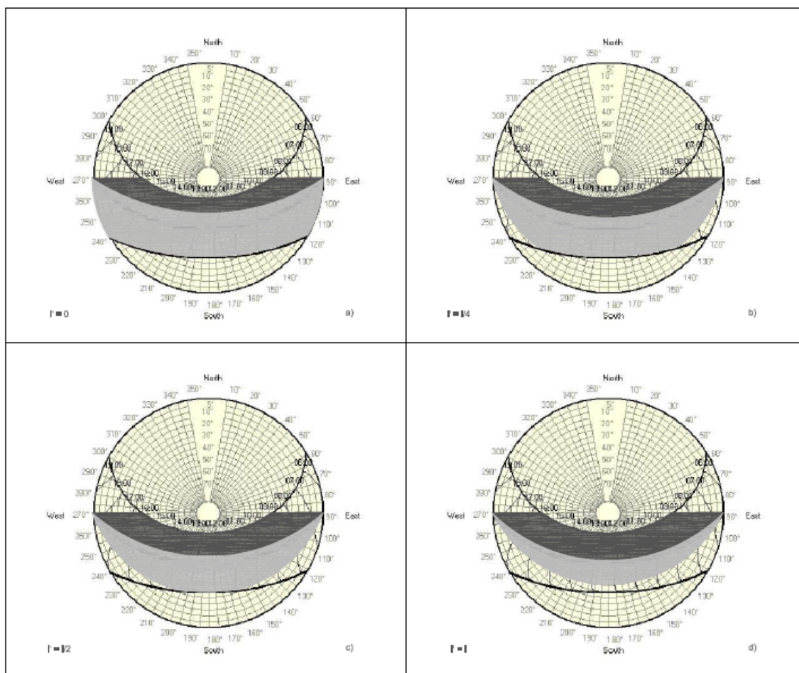
Figura 5. Máscaras de sombra para o vão orientado a sul, \alpha=45^\circ
