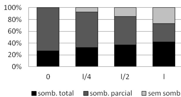
Figura 6. Percentagem da área da máscara de sombra, para diferentes valores de l' ( \alpha=45^\circ )
