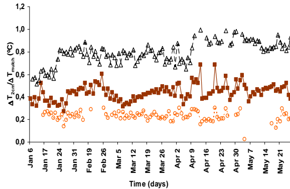
Figure 4. Ratio thermal amplitudes at 2 cm depth/ Thermal amplitudes over mulch: mod B (---△---), mod C (—■—) and mod D (---○---).
