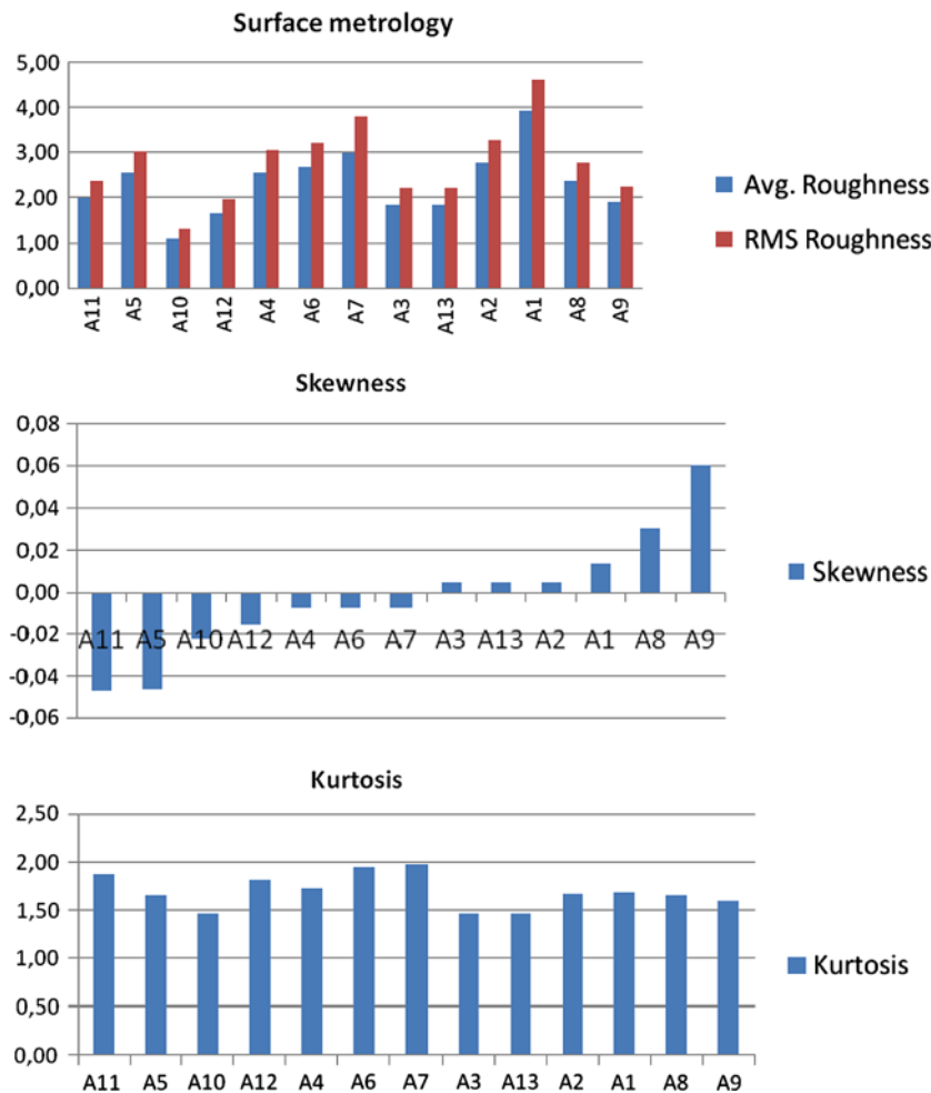
Figure 5. Surface metrology metrics in the 13 sample areas. Figure 5. Surface métrologie métriques aux 13 zones d'échantillon.
