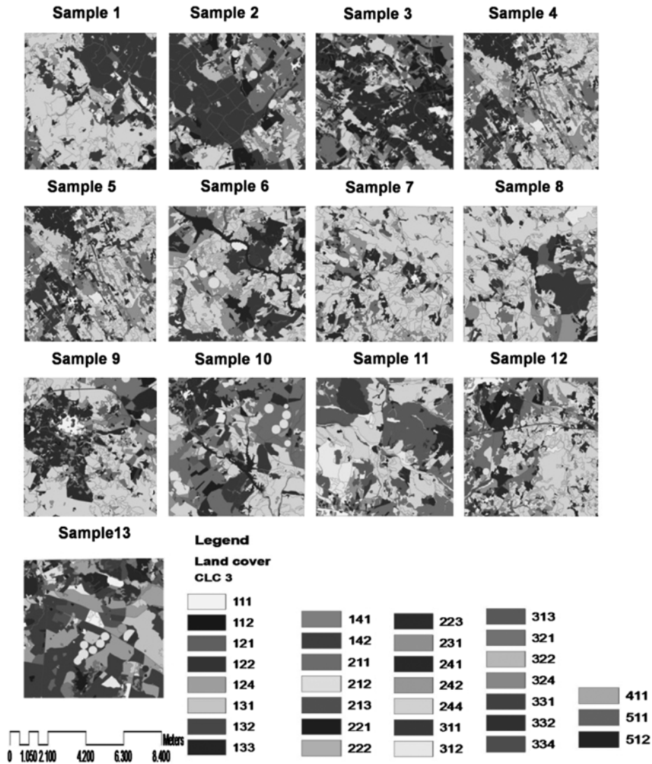
Figure 2. Sample areas local landscape units. Figure 2. Zones d'échantillons des unités locales du paysage.
