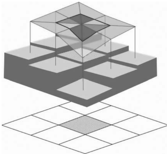
Figure 3. Method to determine true surface area and true surface perimeter of patches. (Figure redrawn according to Jenness 2004 by Hoehstetter et al. 2008). Figure 3. Méthode pour déterminer l'area réelle de la surface et le périmètre réelle de la surface des taches. (Figure redessiné selon Jenness 2004 par Hoehstetter et al. 2008).
