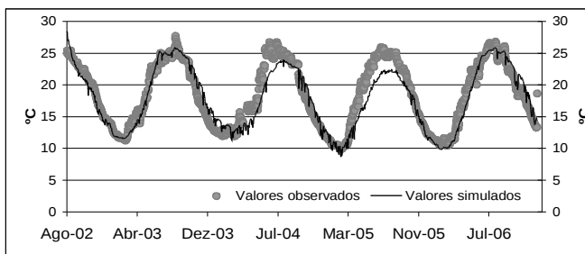
Figura 1 - Evolução da temperatura média observada e simulada à profundidade de 1 metro. Topo: albufeira da Bravura Fundo: albufeira de Alqueva (Evolution of daily water temperature, 1 meter deep, for Bravura and Alqueva reservoirs)
