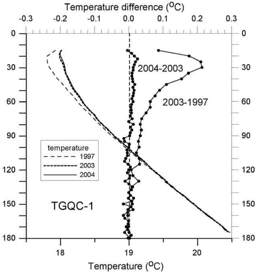
Fig. 1 – Three temperature logs (solid lines and dashed lines) obtained in March 1997, November 2003, and November 2004 in the TGQC-1 borehole. The dotted lines represent the difference of temperatures between the 2003-1997 and 2004-2003 temperature logs. Fig. 1 – Três diagramas de temperatura (linhas a cheio e a tracejado) obtidas no furo TGQC-1 em Março de 1997, Novembro de 2003 e Novembro de 2004. As linhas ponteadas representam a diferença de temperatura entre 2003-1997 e entre 2004-2003.
