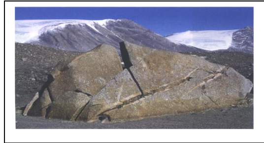
Figura.9 - Crioclastia
