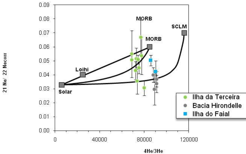
Fig. 1. Projeção num diagrama ^4\text{He}/^3\text{He} versus ^{21}\text{Ne}/^{22}\text{Ne}_{\text{corr}} dos dados obtidos para a ilha da Terceira, do Faial e bacia Hirondele. SCLM: Sub-continental Lithospheric Mantle (Hopp et al., 2004).
