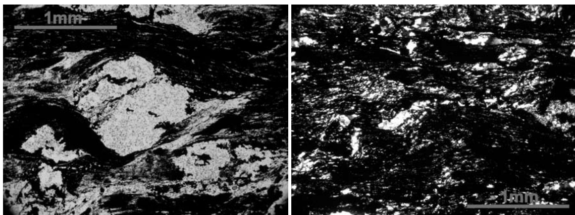
Fig. 8 Fotografias ao microscópio petrográfico em nicóis paralelos (esquerda) e nicóis cruzados (direita) da amostra LJ8.03 (metalidito).
