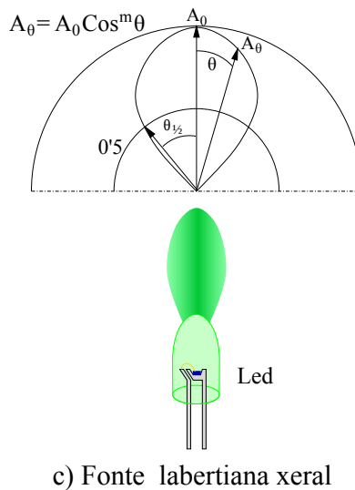
Figura 4: Perfís de radiación típicos
