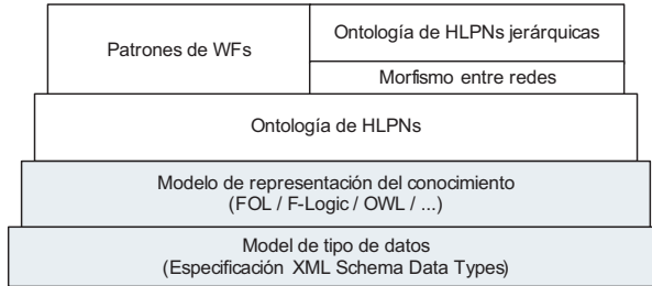
Figura 5.1: Pila de ontologías que da soporte a la representación del modelo de control
