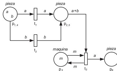
Figura 3.5: Arcos anotados mediante multiconjuntos
