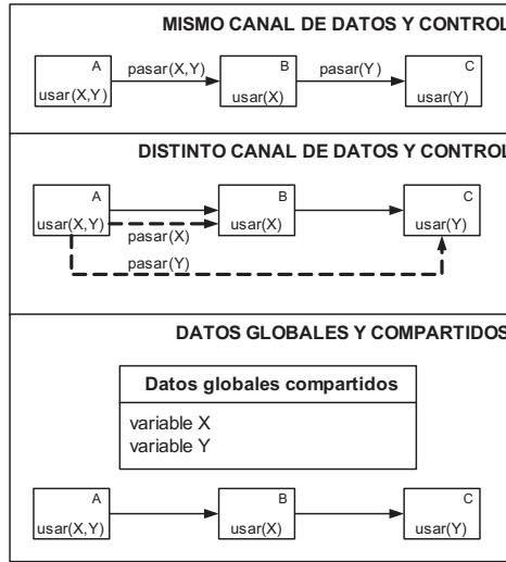
Figura 2.10: Patrón de interacción entre dos tareas
