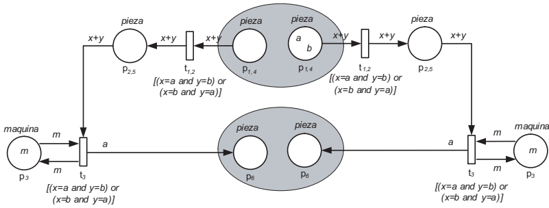
Figura 3.18: Las dos máquinas modeladas a través de la red de la Figura 3.13 comparten la cinta de transporte mediante dos fusiones, que se representan a través de elipses grises. En este caso, las plazas de entrada y salida de ambas máquinas representan la cinta de transporte.
