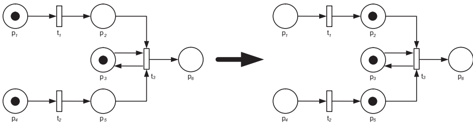
Figura 3.3: Disparo de las transiciones t_1 y t_2
