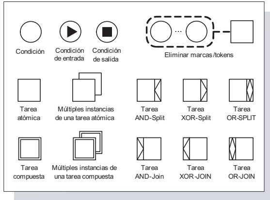
Figura 2.27: Elementos básicos de YAWL
