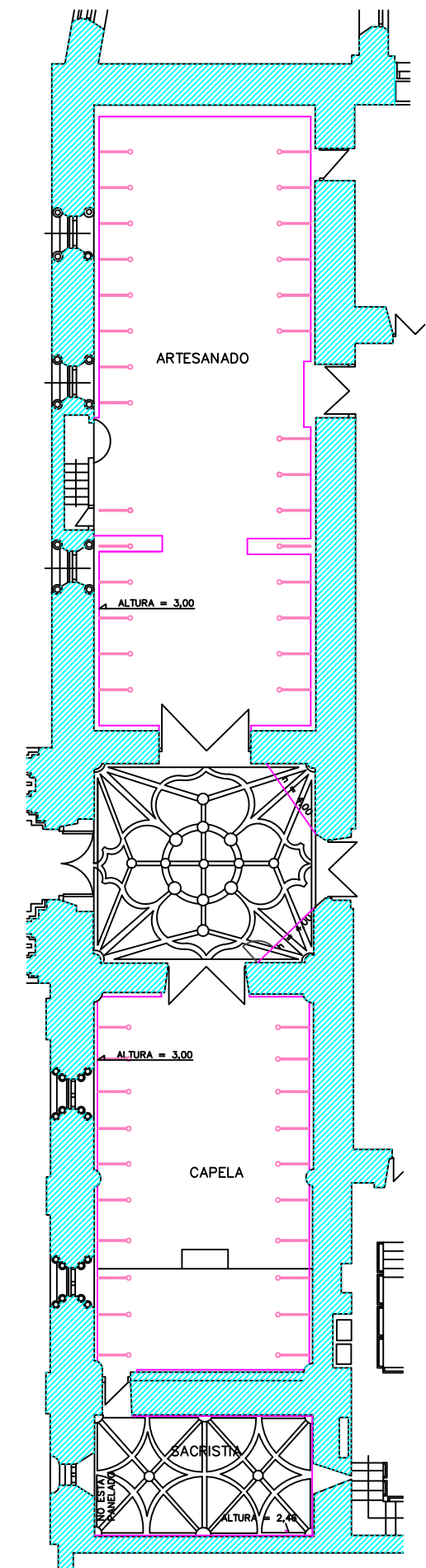
ZONA ARTESANADO E CAPELA Esc: 1/200
