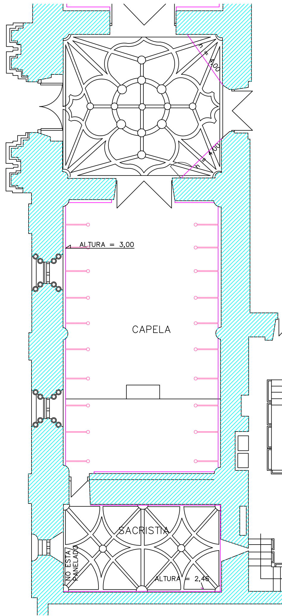
PLANTA BAIXA - ZONA CAPELA - SACRISTÍA Esc: 1/100
