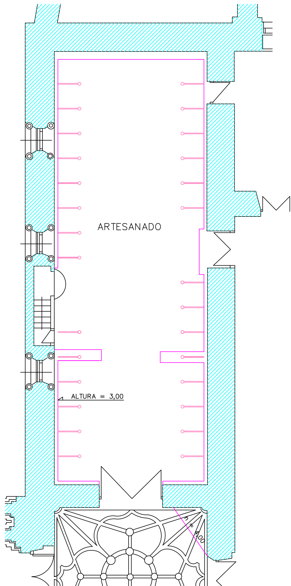
PLANTA BAIXA - ZONA ARTESANADO Esc: 1/100
