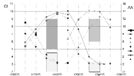
Figura 2.- Digrama de gresificación de las mezclas propuestas. Contracción lineal (CL), capacidad de absorción de agua (AA). Se han sombreado el rango requerido para la obtención de gres rojo no esmaltado (1140-1160°C) y gres porcelánico (1220°-1240°C) en relación con CL (gris oscuro) y AA (gris claro)
