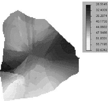
Fig. 6.-Mapa de estimación para el contenido en arena en el nivel 0-15 cm.
