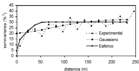
Fig. 3.-Semivariograma experimental y teóricos para la arcilla 0-15 cm.
