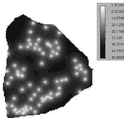
Fig. 8.- Mapa de varianza de los errores de krigado para el contenido en limo en el nivel 0-15 cm.
