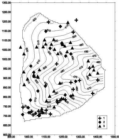
Fig. 1.- Mapa de la cuenca con las curvas de nivel y los puntos de muestreo (1: toma de muestras en el nivel 0-15 cm; 2: en el nivel 0-15 y 15-30; 3: en el nivel 0-15 cm, 15-30 cm y 30-45 cm).
