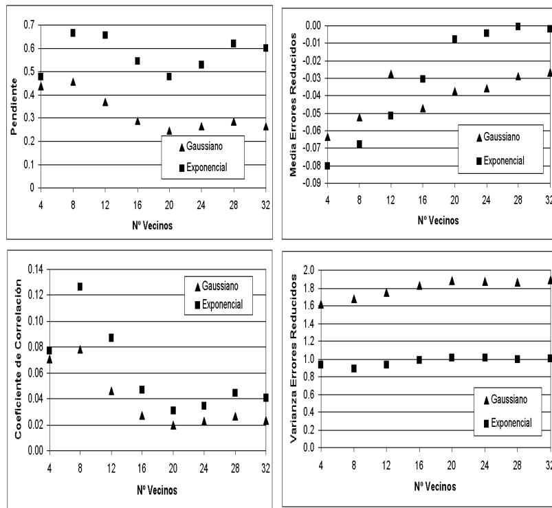
Fig. 4.-Resultados del jack-knifing de los semivariogramas exponencial y gaussiano del contenido en gravas del nivel 0-15 cm.
