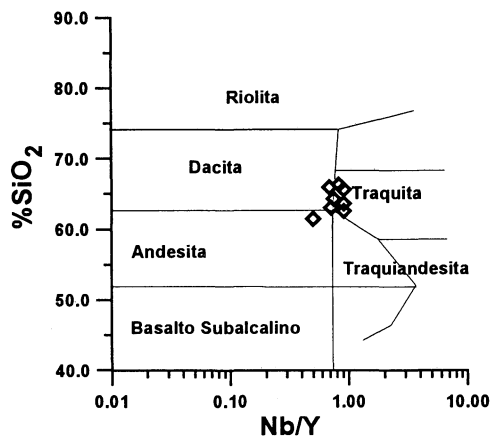
Fig. 8. % SiO 2 -Nb/Y
