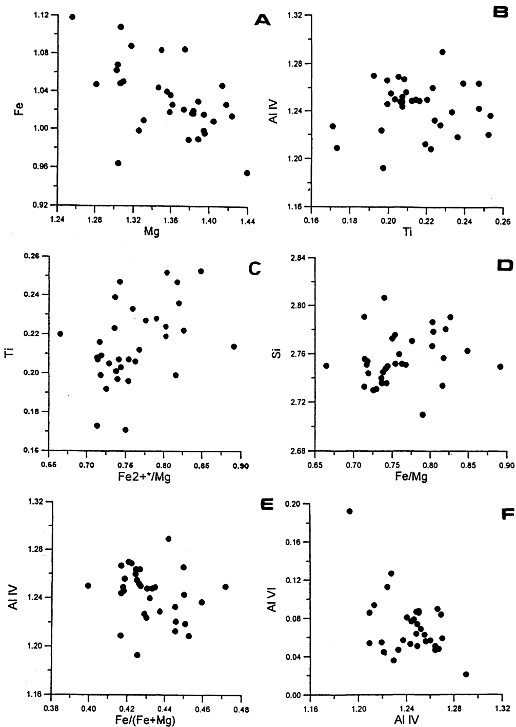
Fig. 7. Relaciones catiónicas en biotitas (Análisis en Tabla 2).
