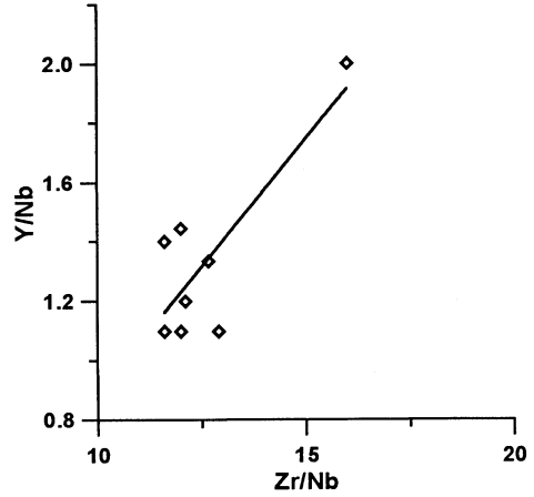
Fig. 11. Relación Y/Nb-Zr/Nb
