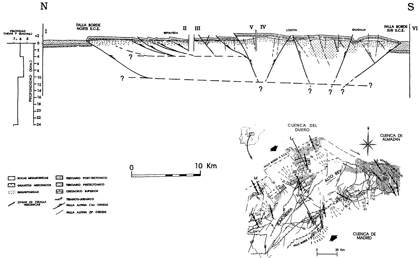
Fig. 2. A) Corte geológico del Sistema Central Español. B) Esquema estructural. Modificado de De Vicente et al. (b), en prensa. Las velocidades sísmicas por debajo del SCE de Suriñach, 1988.
