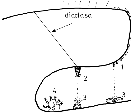
Figura nº 1: Esquema de la formación de los depósitos tipo espeleotema en una cavidad granítica abierta: (1) Estalactita de borde. (2) Estalactita de goteo. (3) Estalagmita. (4) Espeleotemas erráticos. ( de Vidal Romani, J.R., 1983).
