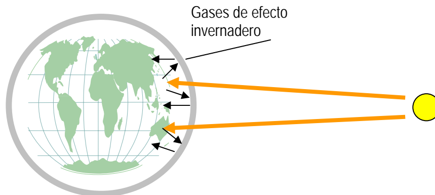
Figura 1. El efecto invernadero debido a la radiación solar y retención del calor en las capas altas de la atmósfera
