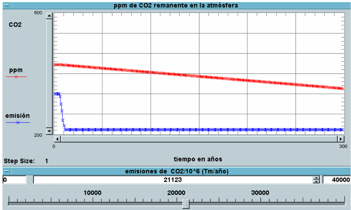
Fig. 2. Evolución del dióxido de carbono en la atmósfera como consecuencia de una reducción de emisiones del 30%
