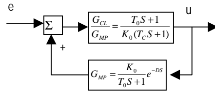
Figura 4. Regulador IMC
