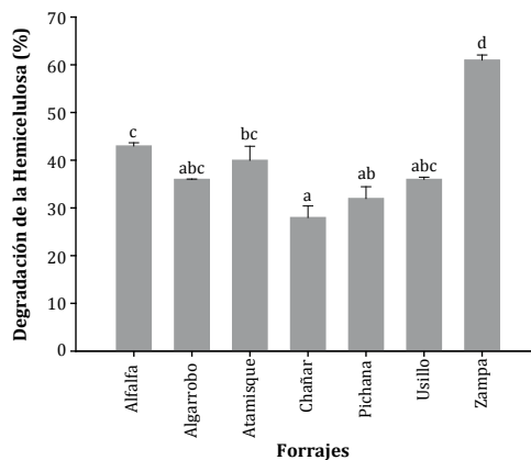
Figura 1. Degradación de la hemicelulosa contenida en el heno de alfalfa y en diversas forrajerías nativas por la cepa P. xylanivorans 2. Las especies forrajerías nativas analizadas fueron: Medicago sativa (alfalfa), Prosopis flexuosa (algarrobo), Capparis atamisquea (atamisque), Geofroea decorticans (chañar), Mimosa ephedroides (pichana), Tricomaria usillo (usillo) y Atriplex lampa (zampa). Letras distintas por encima de las barras indican diferencias estadísticamente significativas ( p < 0,05 ).
