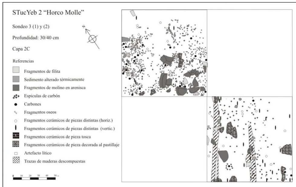
Figura 7. Sondeo 3: horizonte 2C superpuesto a la superficie de ocupación.
