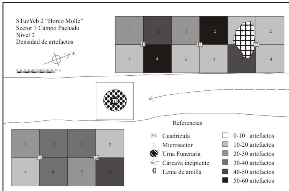
Figura 8. Sector 7: densidad de artefactos, horizonte 2A.
