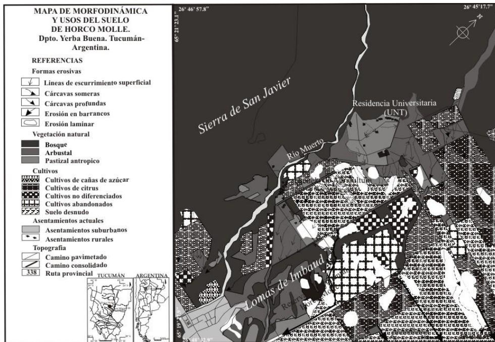
Figura 3. Mapa de morfodinámica y usos del suelo de la localidad de Horco Molle.
