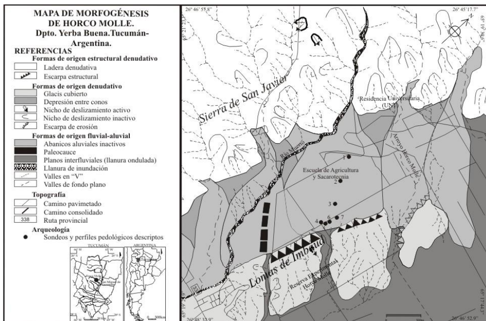
Figura 2. Mapa de morfogénesis de la localidad de Horco Molle.
