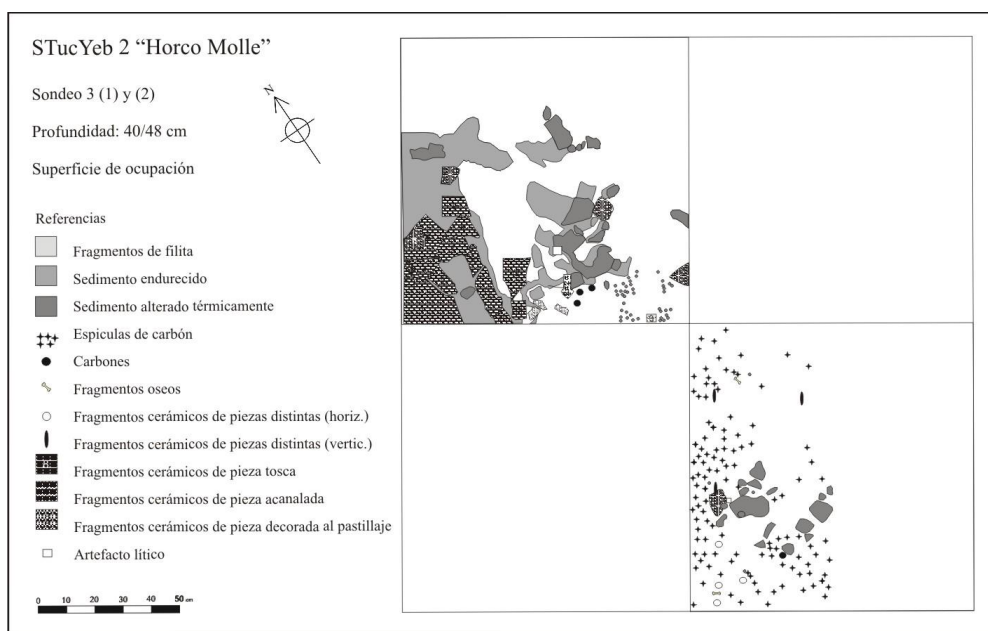
Figura 6. Sondeo 3: superficie de ocupación.
