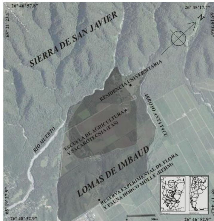
Figura 1. Sitio STucYeb 2 “Horco Molle” (área en gris claro) y abanico aluvial del río Muerto (área en gris oscuro).
