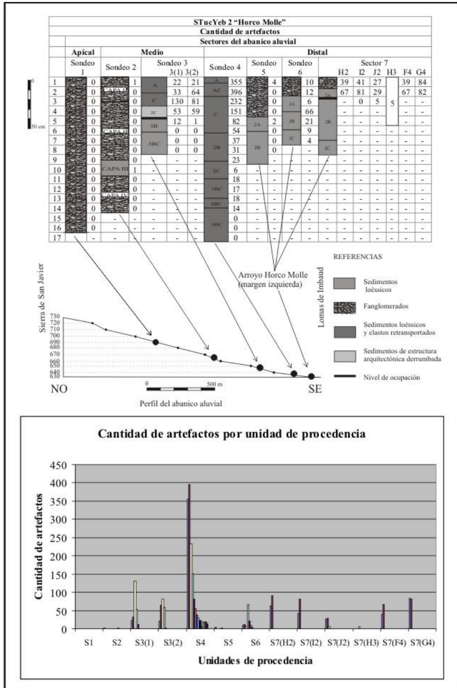
Figura 5. STucYeb 2 “Horco Molle”, abanico aluvial del río Muerto: cantidad y distribución vertical de artefactos para los sectores excavados antedichos, excepto en los niveles con evidencias de ocupación donde se determinaron concentraciones de artefactos de origen conductual.
