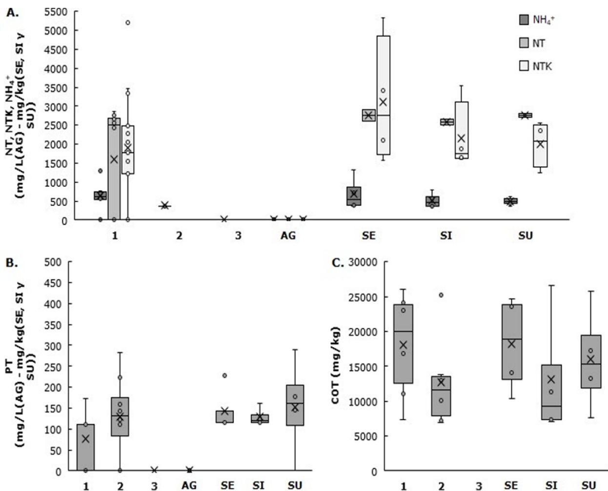
Figura 4. Distribución del contenido de nutrientes considerando los momentos de muestreo y las zonas de la Transición Acuático Terrestre. A. NT: Nitrógeno total, NTK: Nitrógeno total Kjeldahl, NH 4 + : Nitrógeno amoniacal. B. PT: Fósforo Total. Y C. COT: Carbono Orgánico Total.
