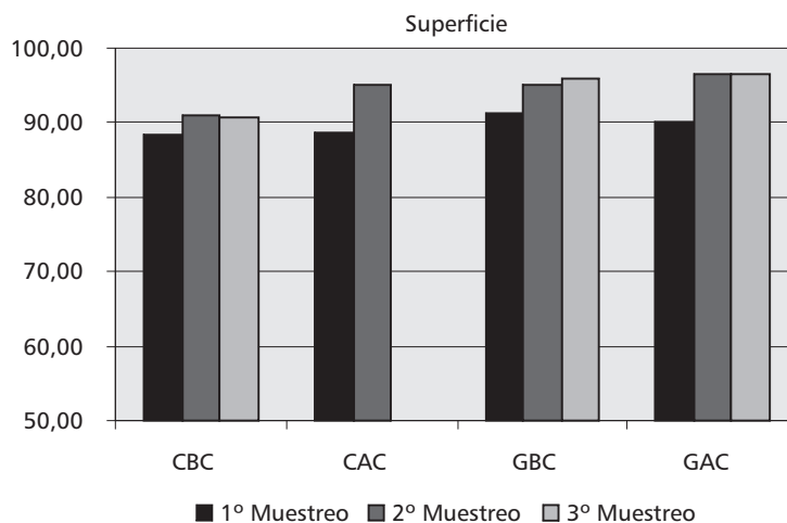
Gráfico 2: Compactación relativa (%)
