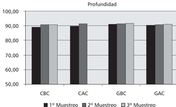
Gráfico 2: Compactación relativa (%)
