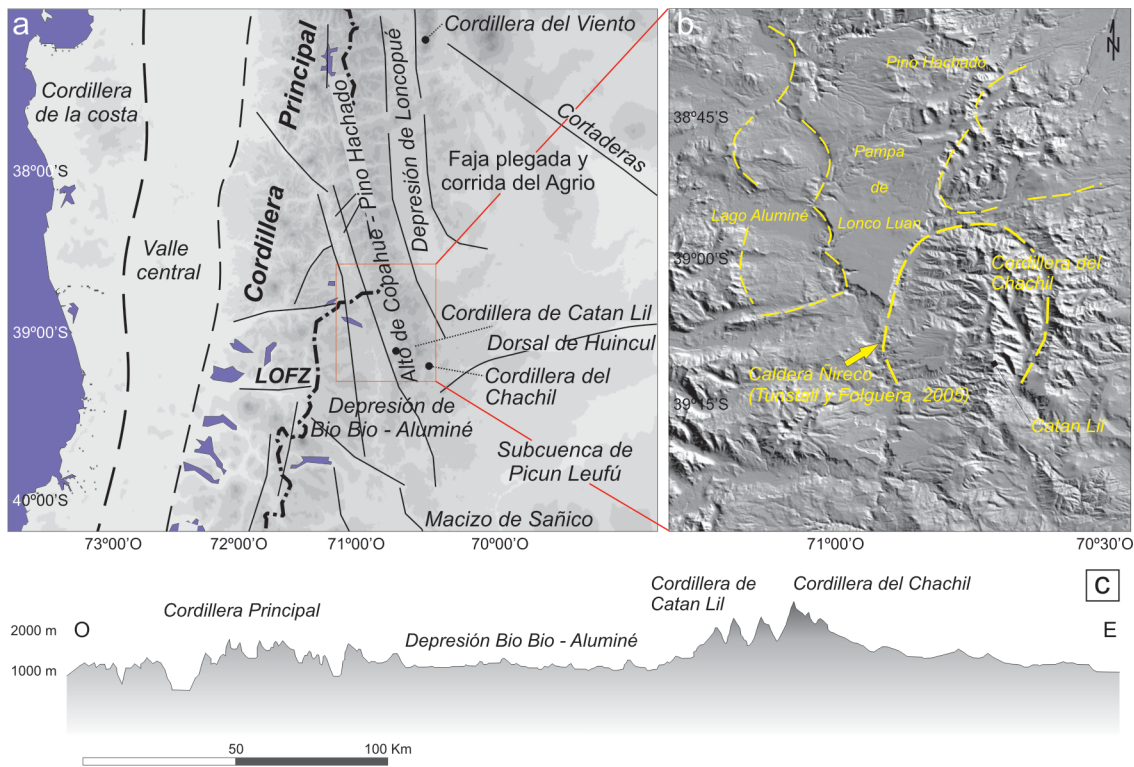
Figura 1: Ubicación del área de estudio: a) Configuración tectónica y principales unidades morfoestructurales de los Andes entre los 37° y 40°S; b) Modelo de elevación digital entre los 38°30' y los 39°30' S. Las trazas discontinuas corresponden a los límites de algunas de las calderas propuestos por Tunstall y Folguera (2005) para la zona; c) Topografía exagerada a lo largo de una transecta este-oeste ubicada a los 39°S.
