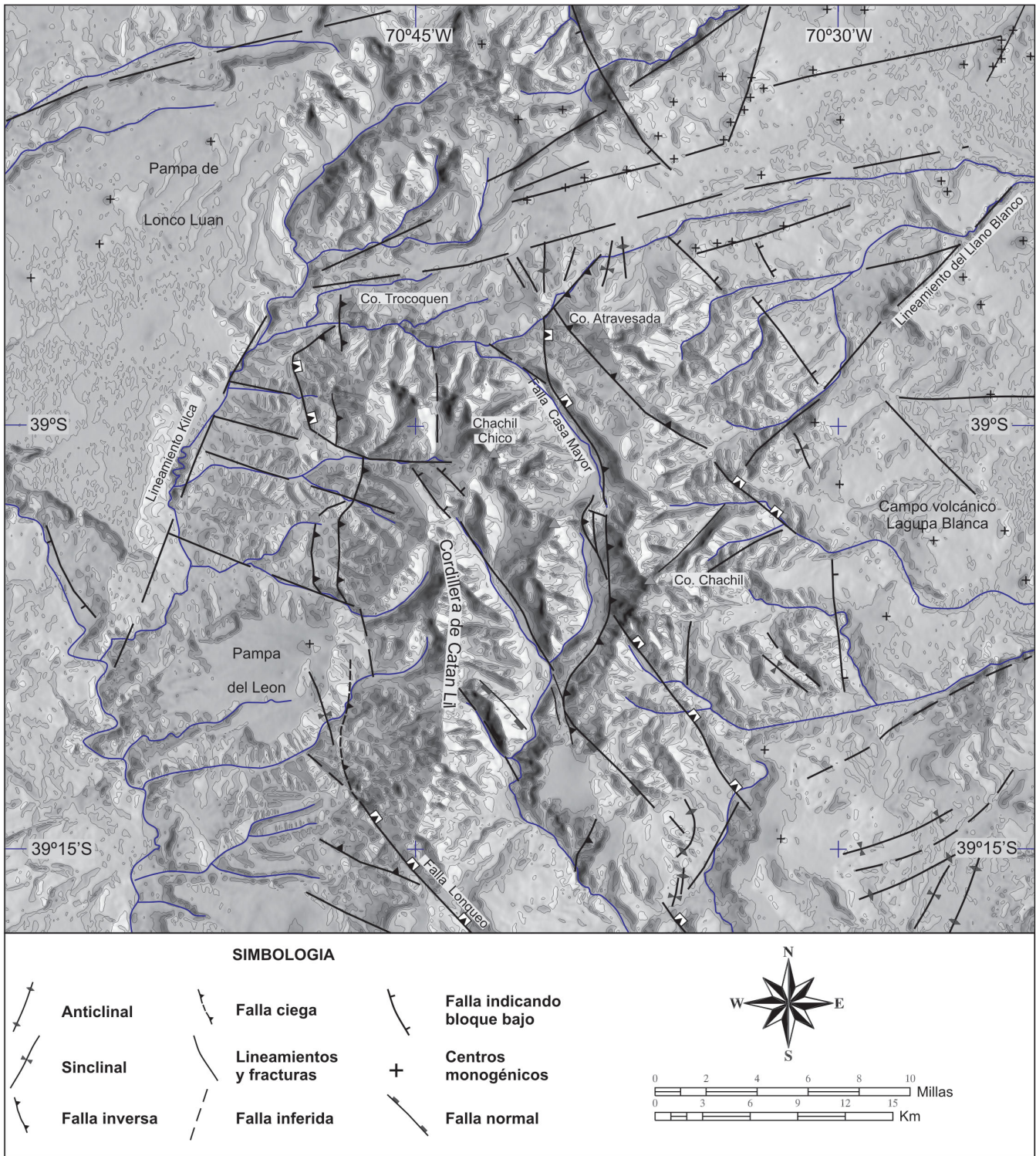
Figura 3: Rasgos morfoestructurales y tectónicos regionales de las cordilleras de Catan Lil, Chachil y áreas aledañas. Modelo de elevación digital, contornos topográficos (equidistancia: 50 m) y mapa estructural sobreimpuesto (Modificado de García Morabito y Ramos 2008, García Morabito 2010 y García Morabito et al. 2010).
