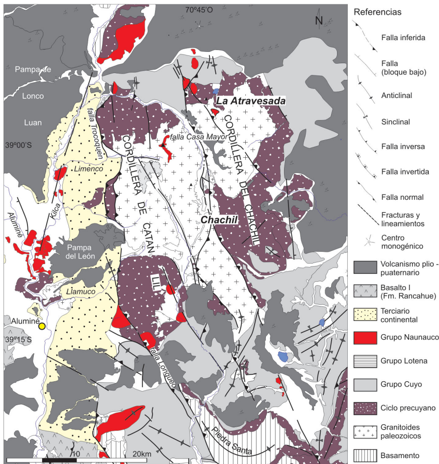
Figura 2: Mapa geológico del área. Geología modificada de Galli (1969), Turner (1973, 1976) y Leanza (1990). Estructura modificada de García Morabito y Ramos (2008), García Morabito (2010) y García Morabito et al. (2010).
