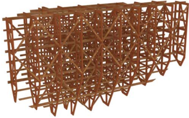
Lâminas Longitudinais
