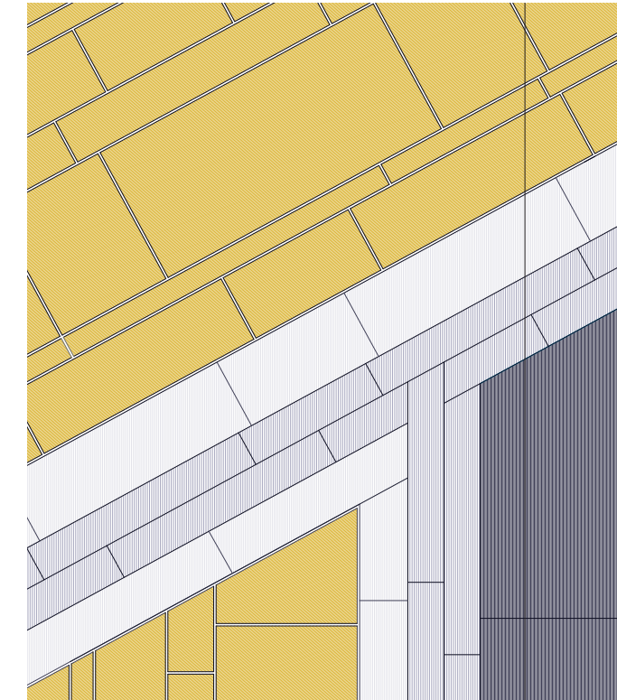
Estereotomia da Praça Praça Caldeira Amarello Lillo escovado
