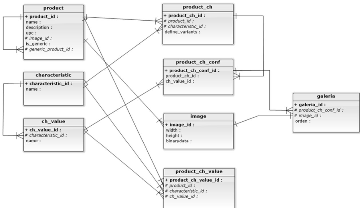
Figura 15. Esquema definitivo de la base de datos de productos
