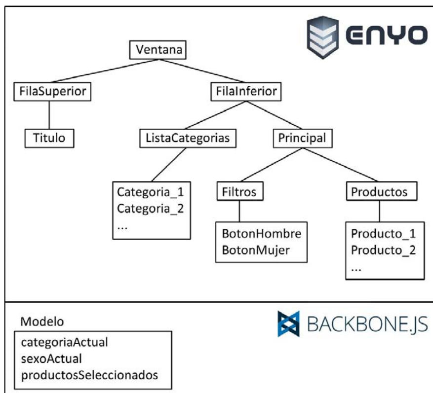
Figura 20. Esquema de componentes de la aplicación cliente
