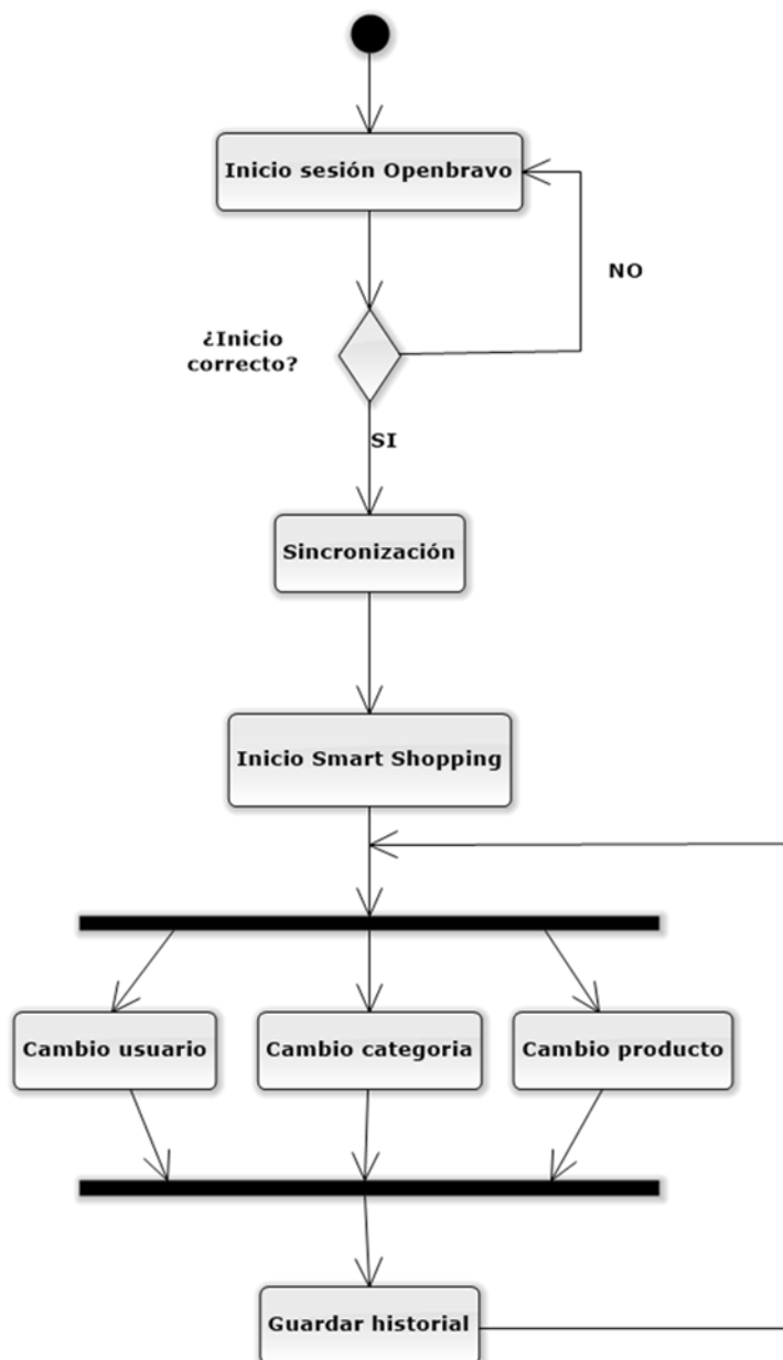
Figura 5. Diagrama de actividades
