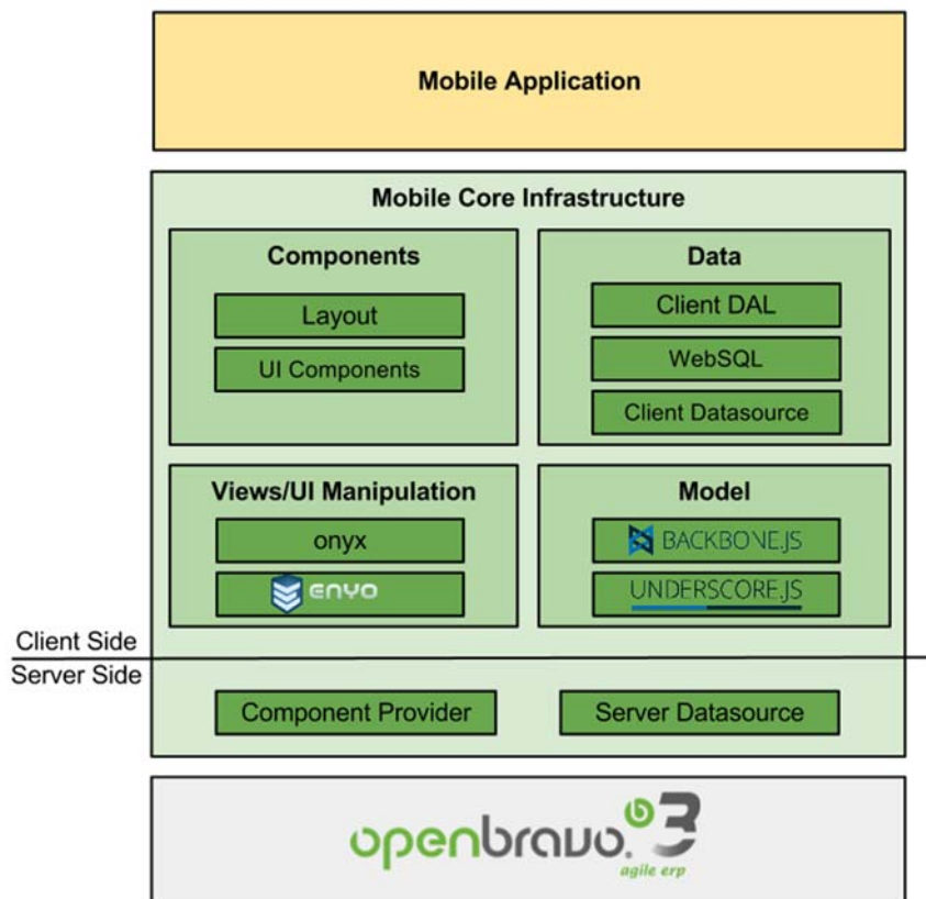
Figura 11. Arquitectura Openbravo Mobile
