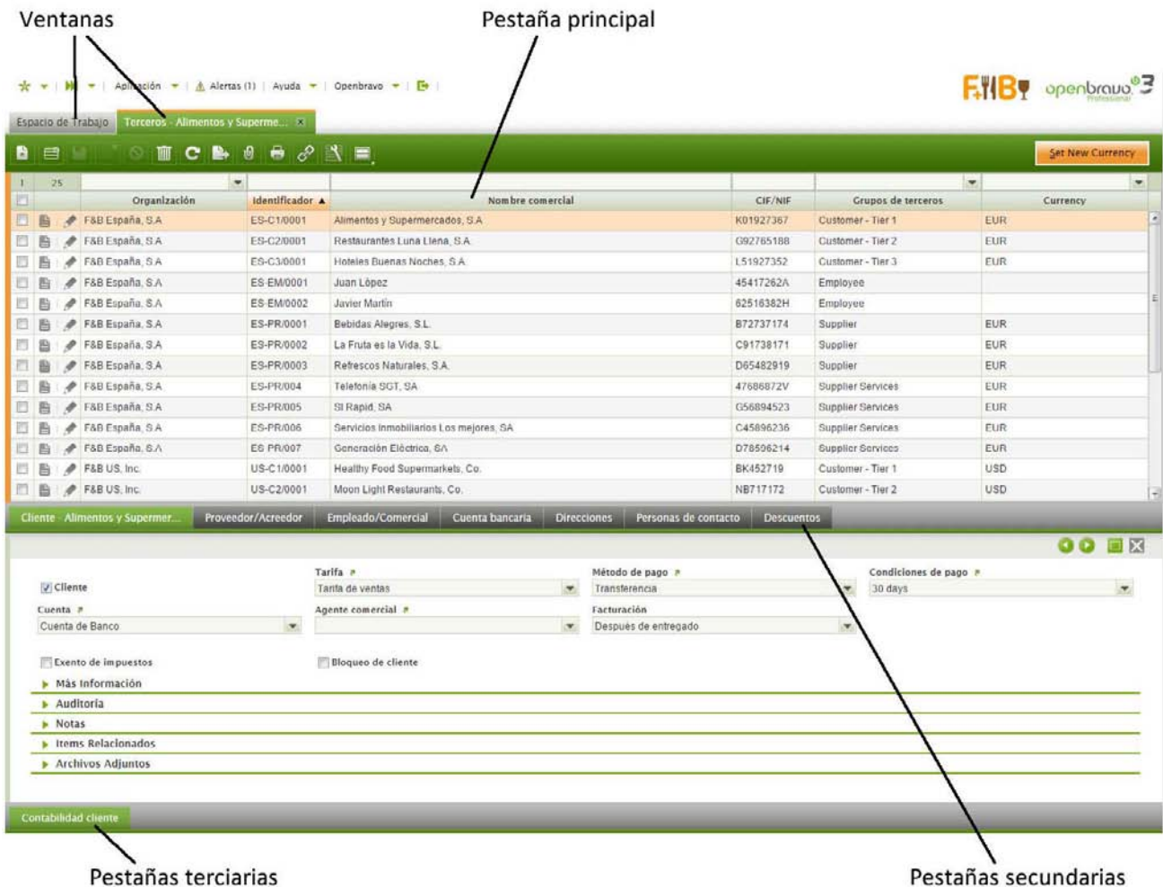
Figura 10. Secciones de la interfaz de Openbravo
