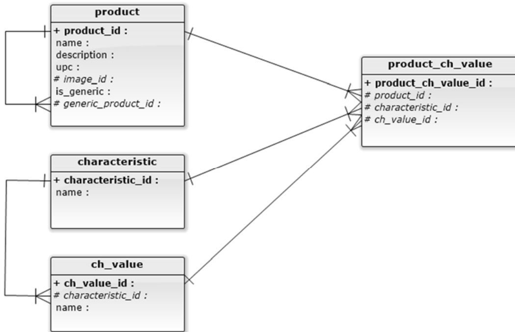
Figura 13. Esquema base de datos variantes de productos
