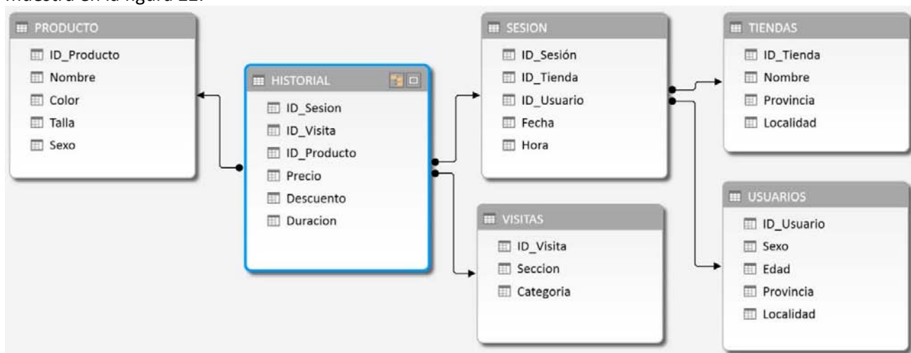
Figura 22. Diagrama en estrella
