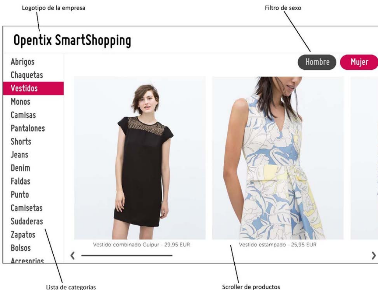
Figura 7. Diseño sección Categorías
