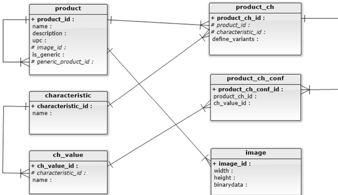
Figura 12. Esquema base de datos productos genéricos
