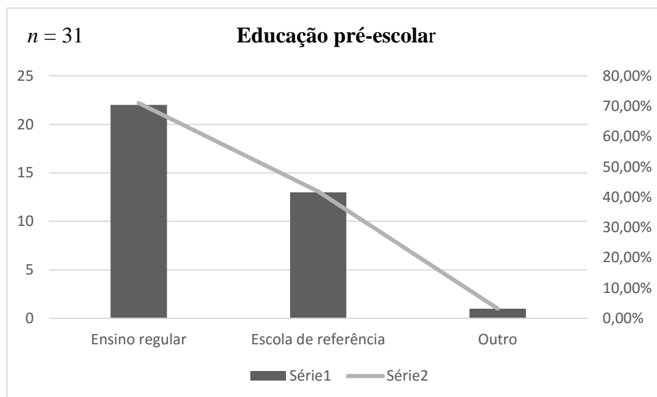
Figura 2.2: Educação pré-escolar
