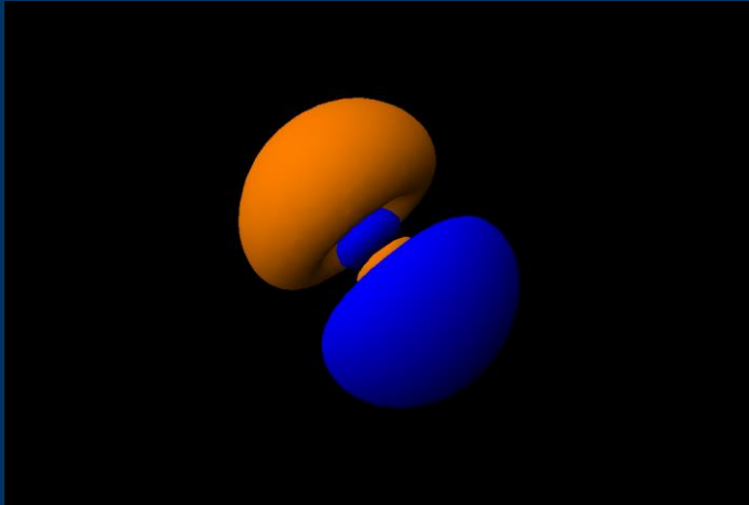
Orbitais 3p e 3d
