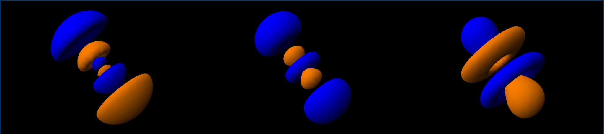
Orbitais 4p, 4d e 4f
