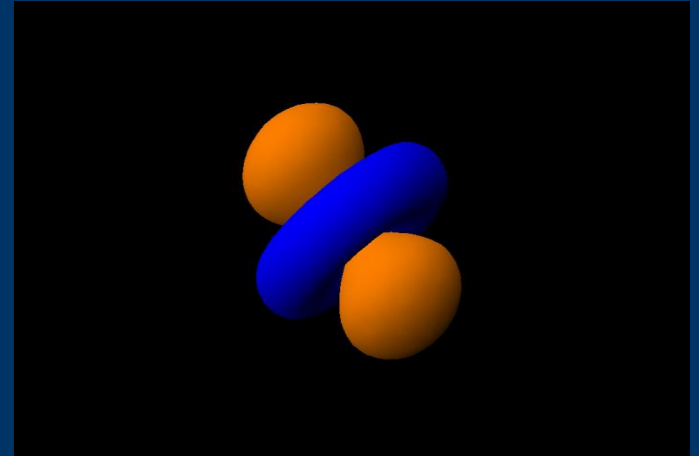
Orbitais 3p e 3d
