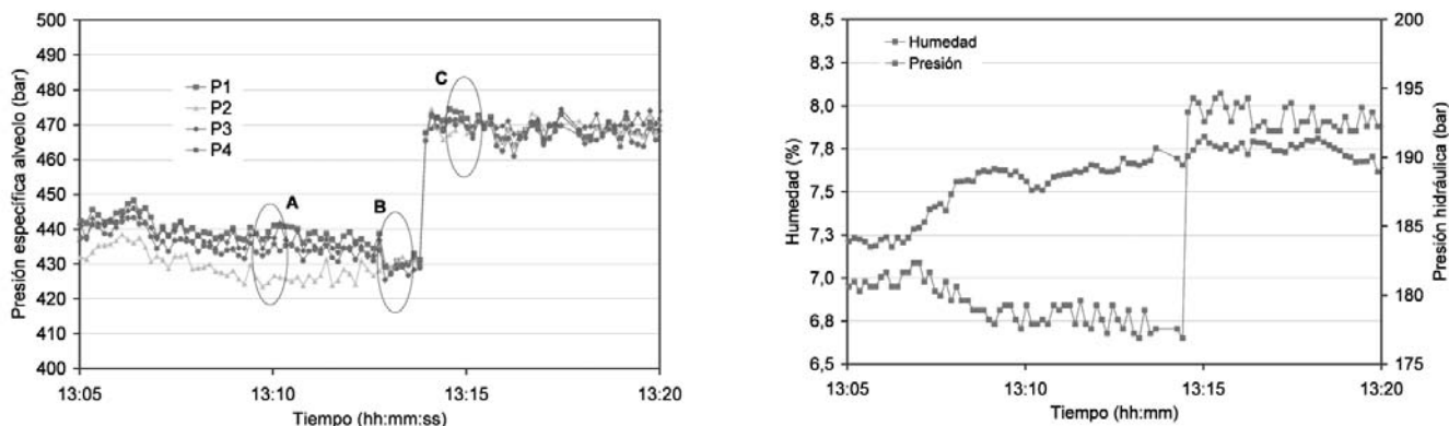
Figura 7. Evolución en el tiempo de las presiones específicas máximas registradas (izq.) y de la humedad del polvo atomizado y la presión en el circuito hidráulico (der.) durante 15 minutos.
