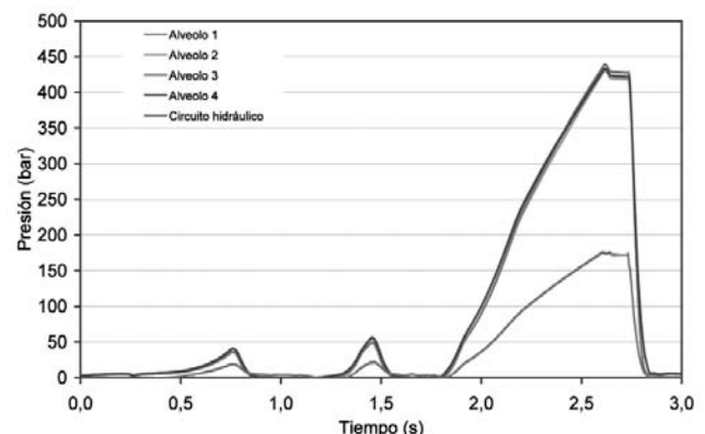
Figura 6. Evolución de las presiones registradas durante un ciclo de prensado sin corrección de la carga (izq.) y un ciclo de prensado con corrección (der.).
