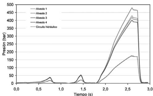
Figura 6. Evolución de las presiones registradas durante un ciclo de prensado sin corrección de la carga (izq.) y un ciclo de prensado con corrección (der.).
