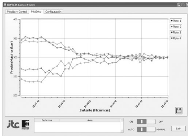
Figura 3. Evolución histórica de las presiones máximas registradas en cada alvéolo.
