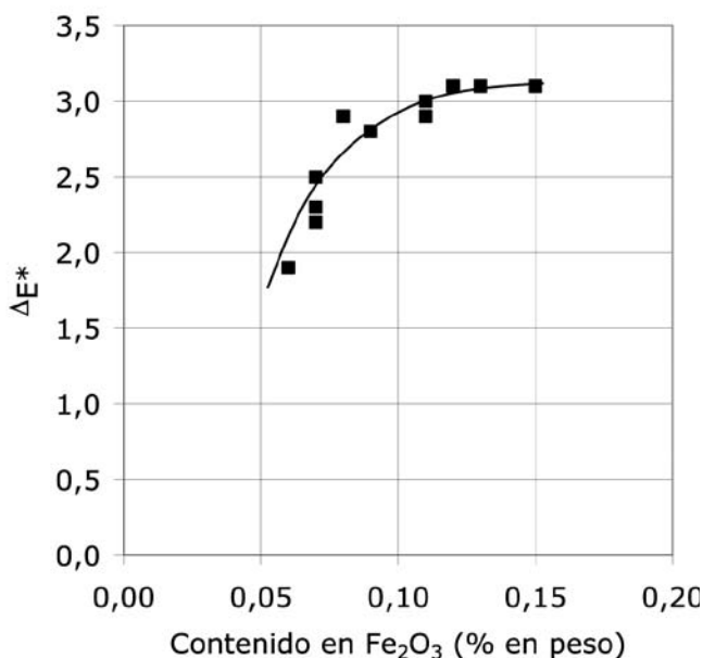
Figura 2. Variación del cambio de color con el contenido en \text{Fe}_2\text{O}_3 de los esmaltes
