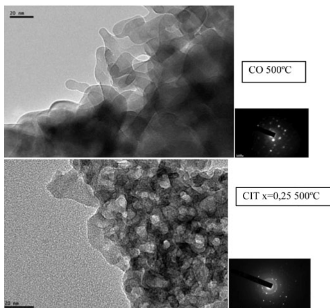
Figura 13. Microscopía MET y difracción de electrones asociada en las muestras indicadas.
