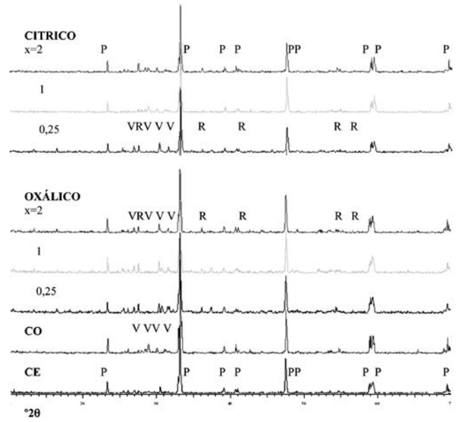
Figura 3. DRX de las muestras V-CaTiO 3 calcinadas a 1000°C/3h: P (perovskita CaTiO 3 ), V (pirovanadato de calcio CaV 2 O 7 ), R (rutilo TiO 2 ).
