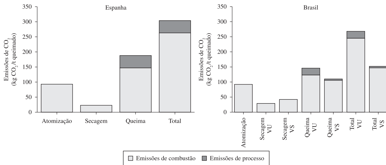
Figura 4. Emissões médias de CO 2 (estado estacionário).
