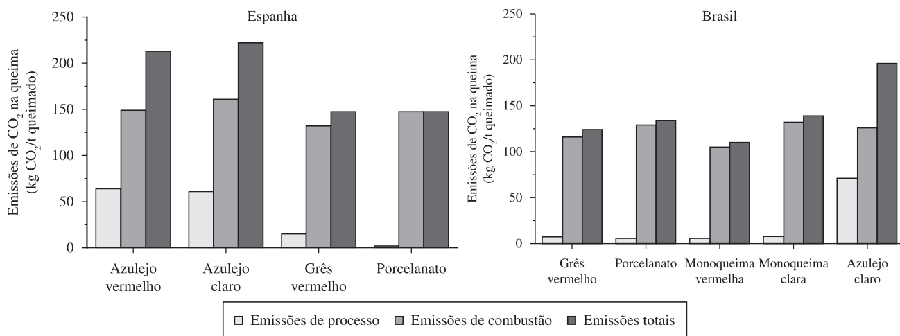
Figura 3. Emissões de CO 2 na etapa de queima (estado estacionário).
