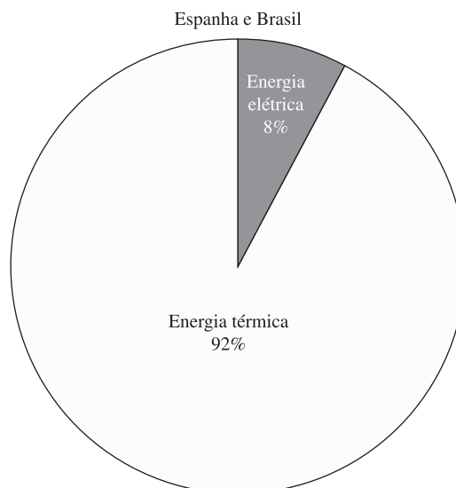
Figura 2. Distribuição de consumos energéticos no setor de fabricação de revestimentos cerâmicos e pó atomizado, durante o ano de 2008 (Espanha) e 2009 (Brasil).
