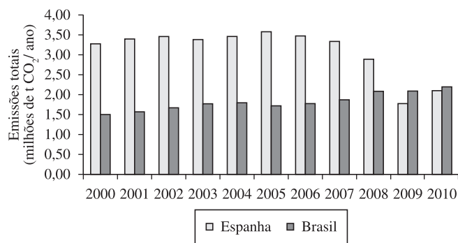
Figura 5. Evolução das emissões setoriais de CO 2 na Espanha e no Brasil.
