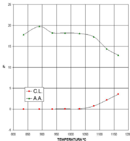
Fig 1. Curvas de gresificación mostrando la variación de la contracción lineal y capacidad de absorción de agua con la temperatura.
