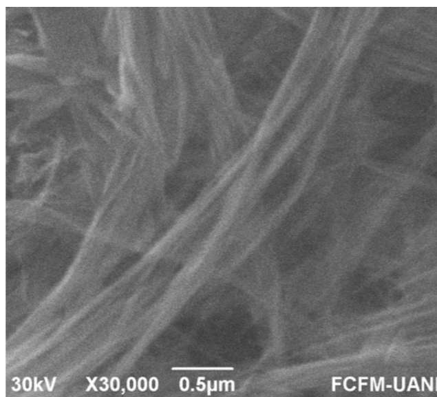
Figura 4. Imágenes SEM de nano alambres de Cu(OH) 2 .
