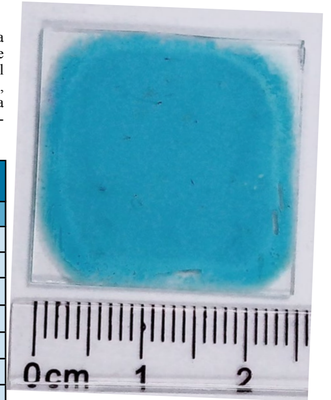
Figura 2. Película de nanoalambres de \text{Cu}(\text{OH})_2 .
