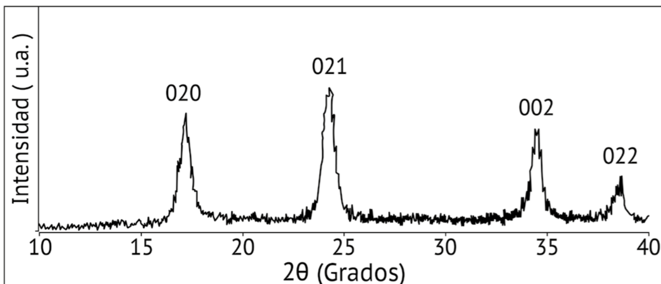
Figura 3. Patrón XRD de nano alambres de Cu(OH) 2 .
