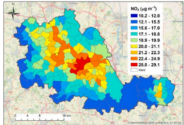
(d) NO 2 for Case Re0.5
