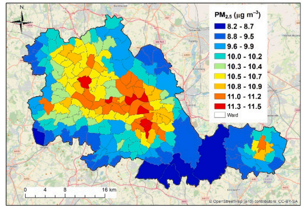
(d) PM 2.5 for Case Re0.5
