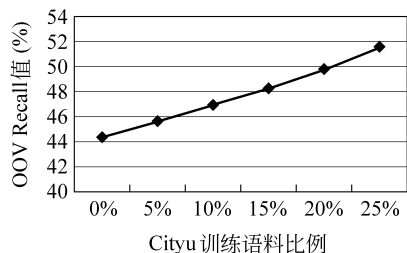
图2 系统在 Cityu 测试语料上面的 OOV Recall 值
