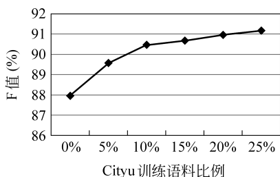
图1 系统在 Cityu 测试语料上面的 F 值
