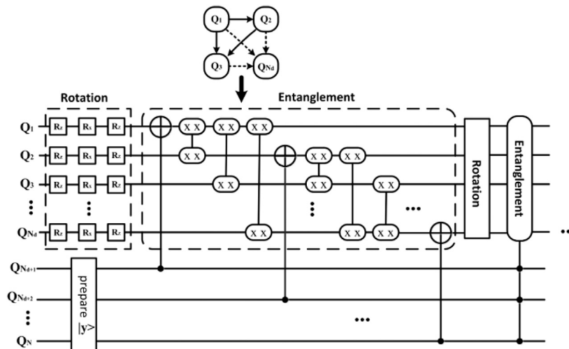
Fig. 24. QGAN quantum circuit generator [48].
