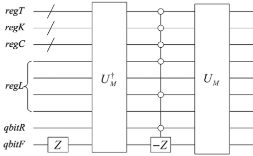
Fig. 17. QDCNN-Net G oracle [43].
