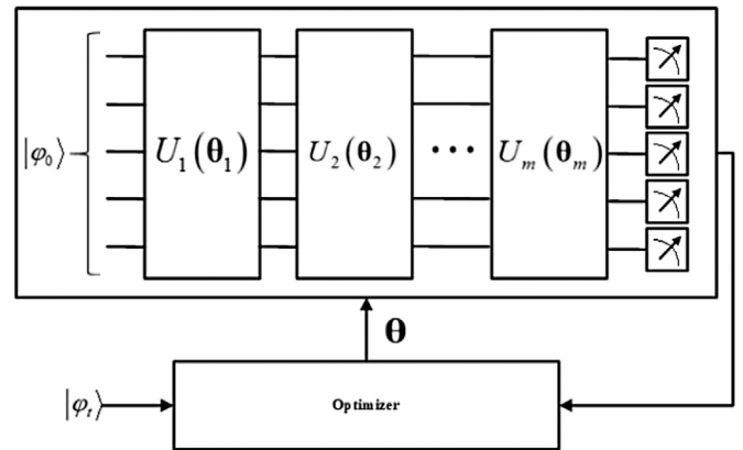
Fig. 3. VQC framework [29].
