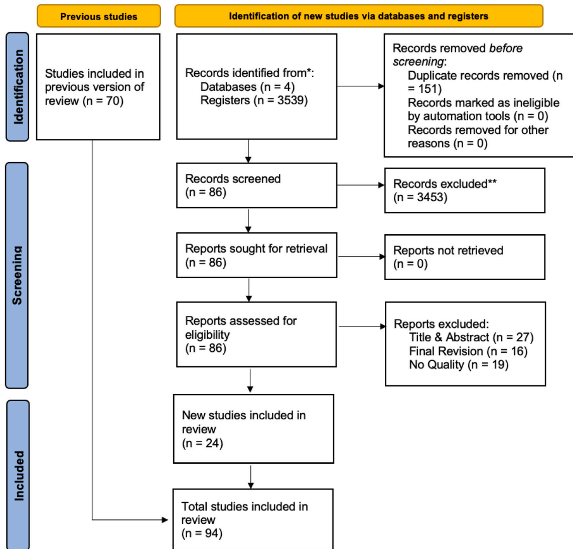
Fig. 2. PRISMA diagram.
