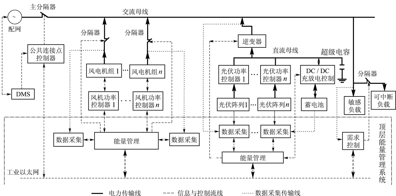
图1 华南理工大学电力学院新能源研究中心风力-太阳能发电系统组成示意图
