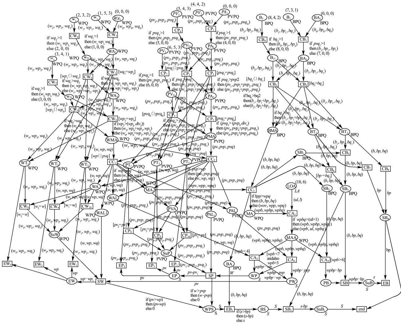
图6 基于有色Petri网的系统能量优化与调度动态过程模拟
