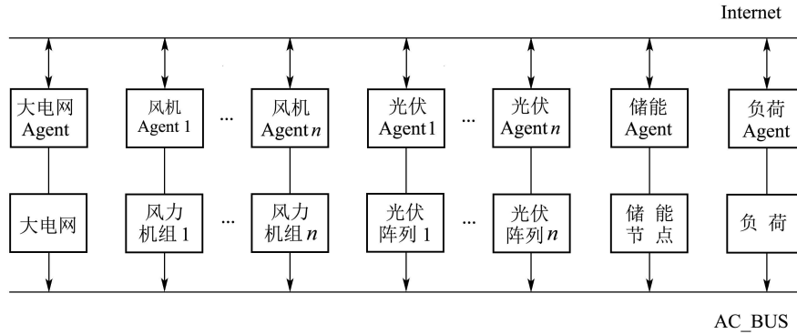
图2 能量管理系统的基本结构图
