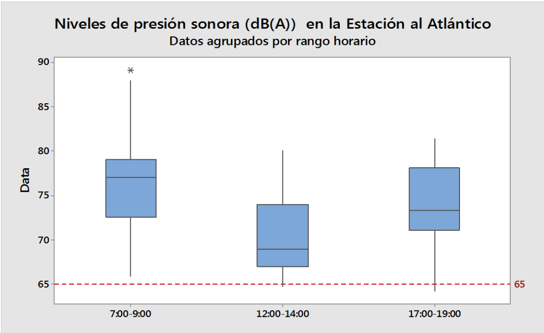
Gráfico 3: Niveles de presión sonora en la Estación al Atlántico
