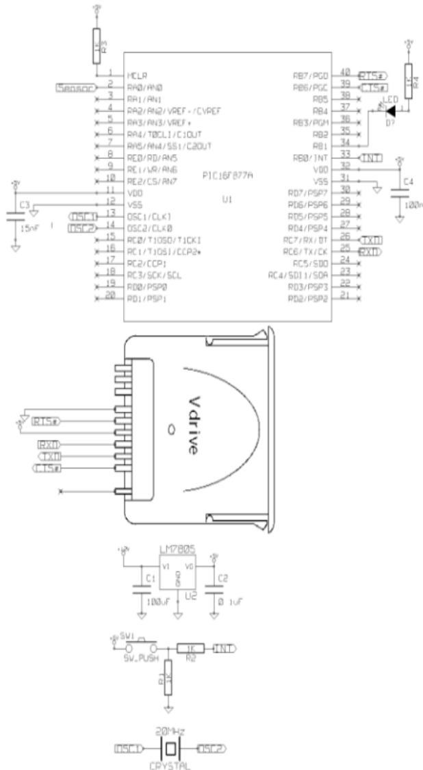
Figura 15: Diagrama de tercer nivel: Componentes
