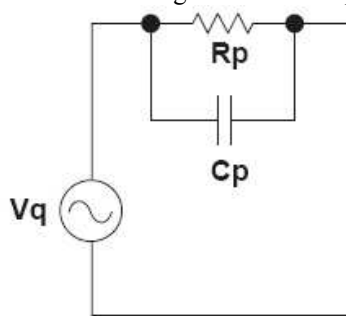
Figura 8. Modelado de voltaje de un sensor piezoeléctrico.
