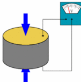
Figura 3. Funcionamiento de un sensor piezoeléctrico.
