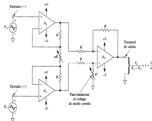
Figura 19. Amplificador de instrumentación utilizado como acondicionador de señal (4).
