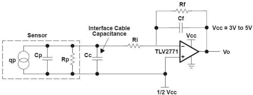
Figura 11. Circuito de un amplificador de carga.
