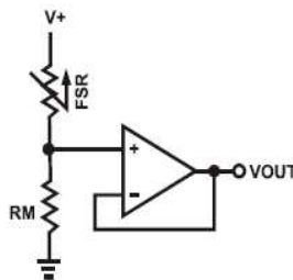
Figura 17. Convertidor de fuerza a voltaje2.
