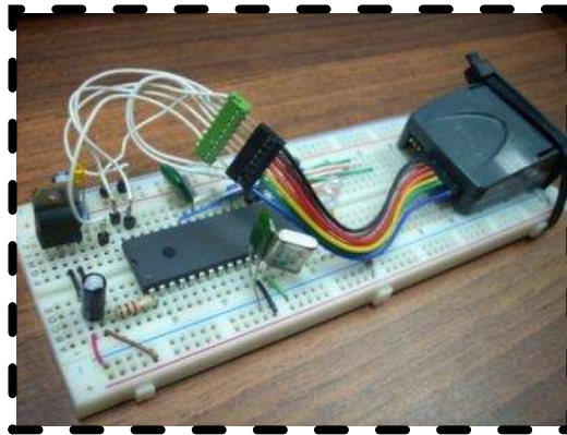
Figura Datalogger
