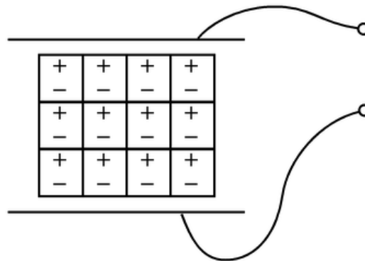
Figura 2. Sensor basado en el efecto piezoeléctrico.
