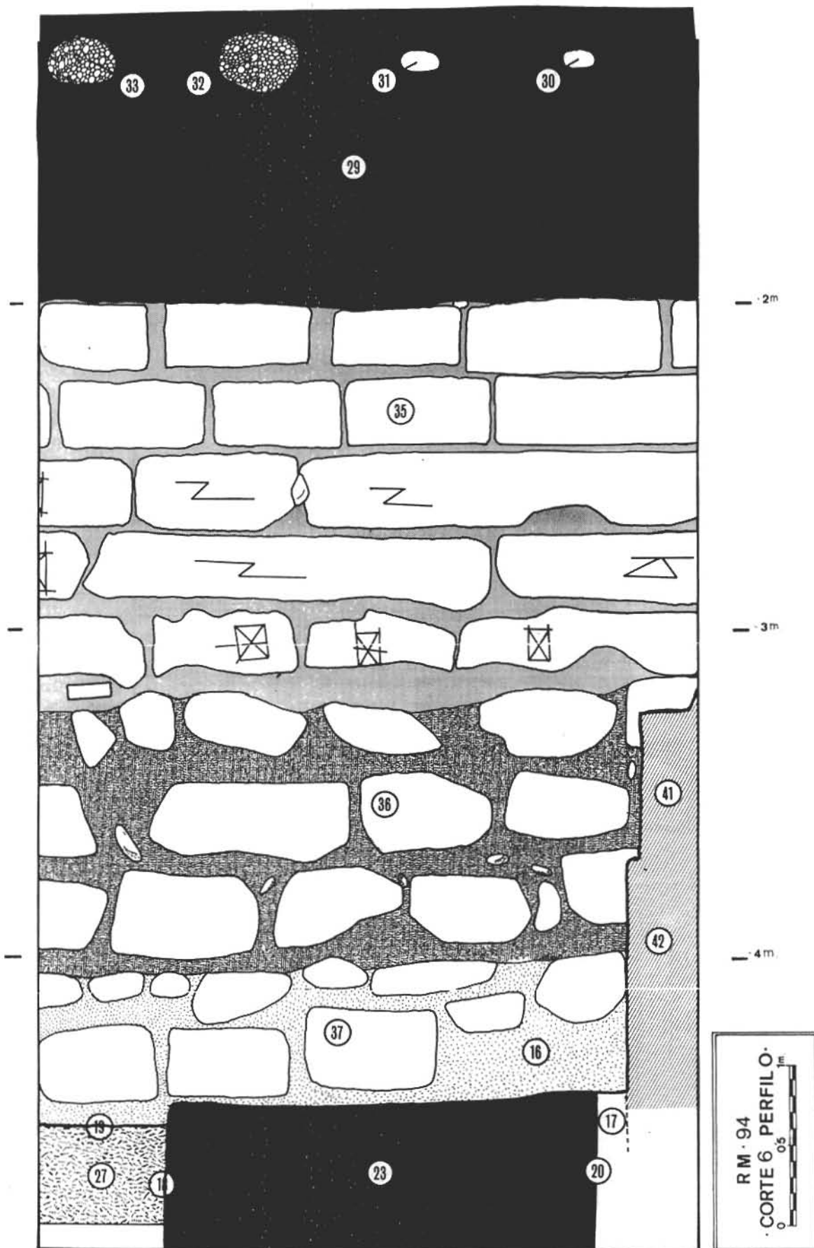
Fig. 9. Cimentación y zócalo de la muralla cristiana a extramuros, documentado en corte 6 (perfil Oeste corte 6)
