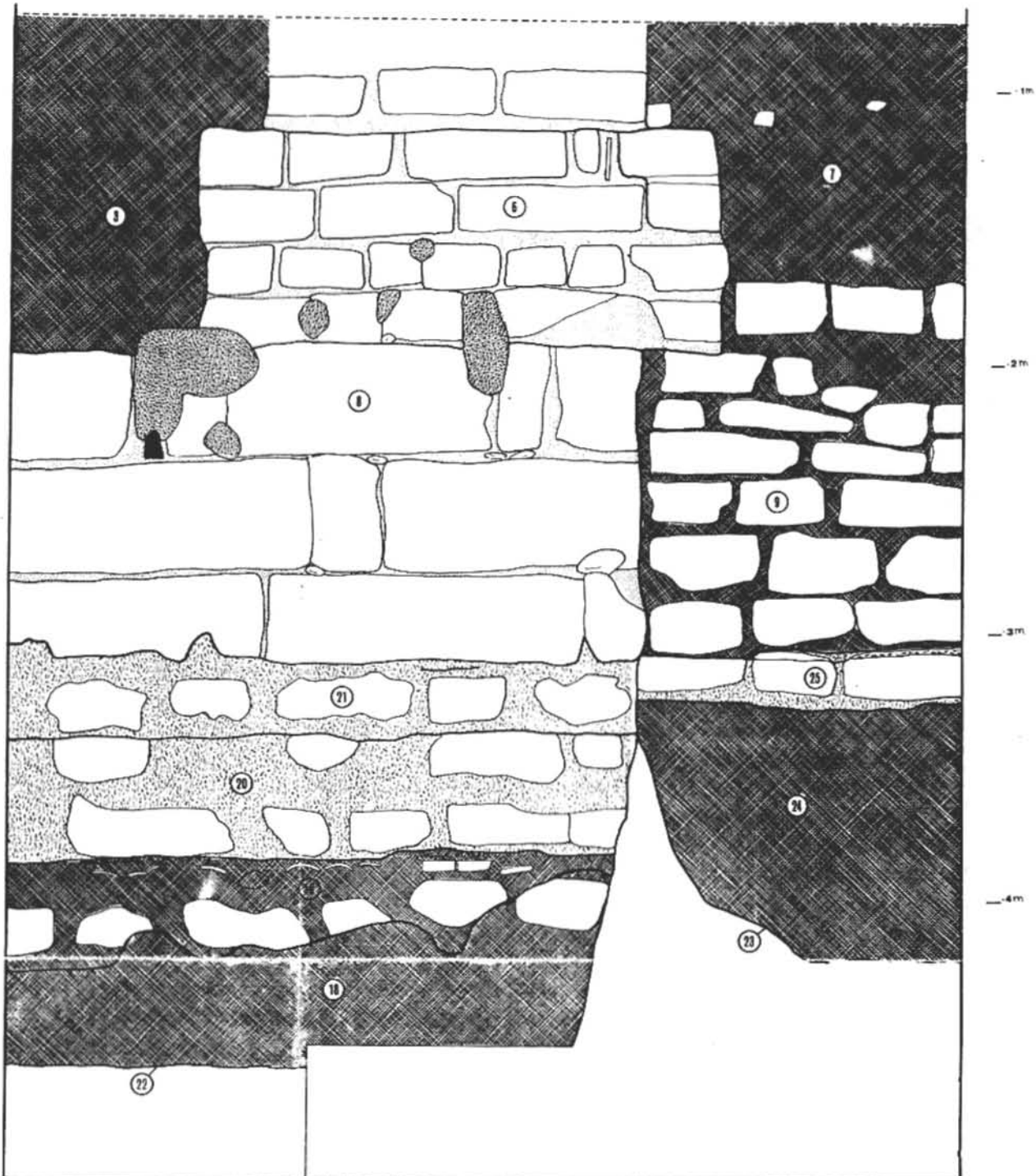
RM-94 CORTE 3 PERFIL E.
