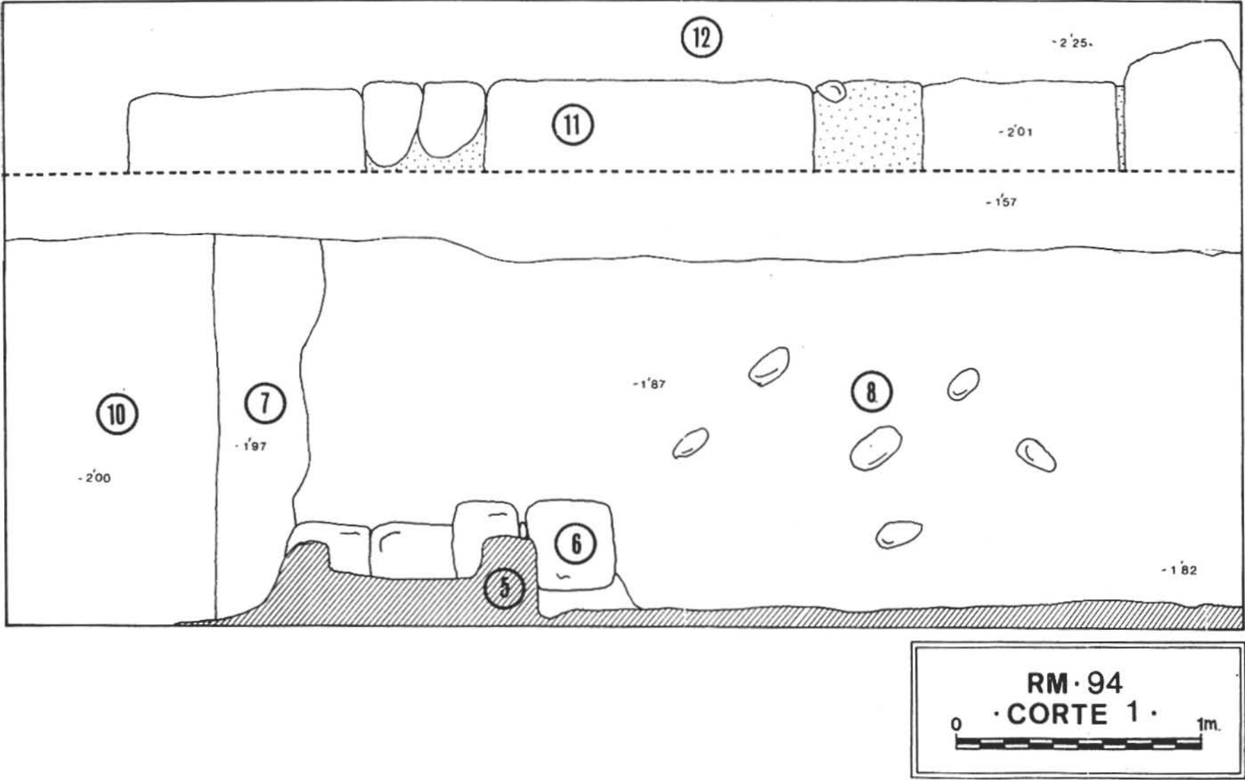
FIG. 12. Elementos relacionados con la antigua escalera de acceso al adarve documentada en el corte 1 (planta final corte 1)
