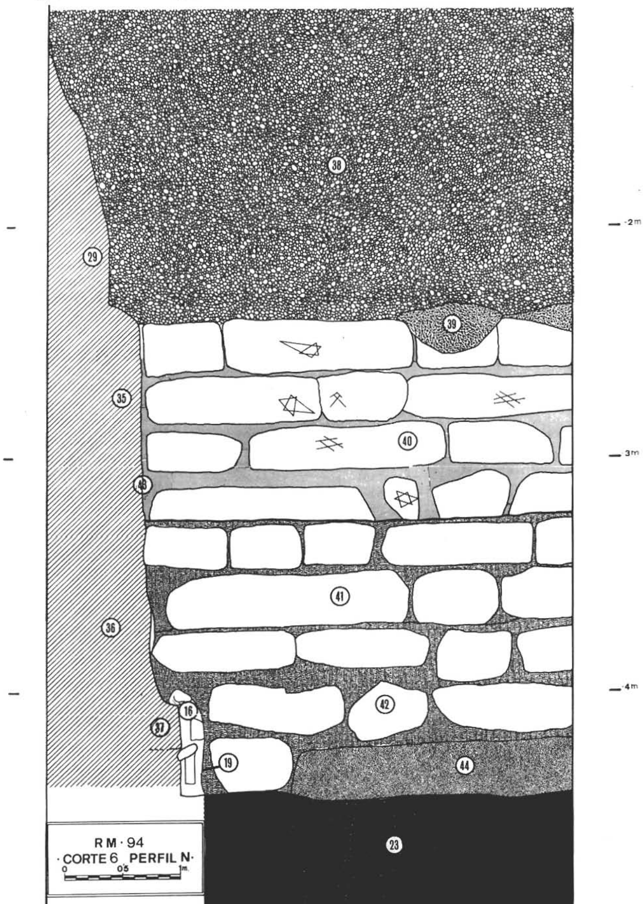
FIG. 10. Cimentación y zócalo de la torre 1 en su cara meridional (perfil Norte corte 6)
