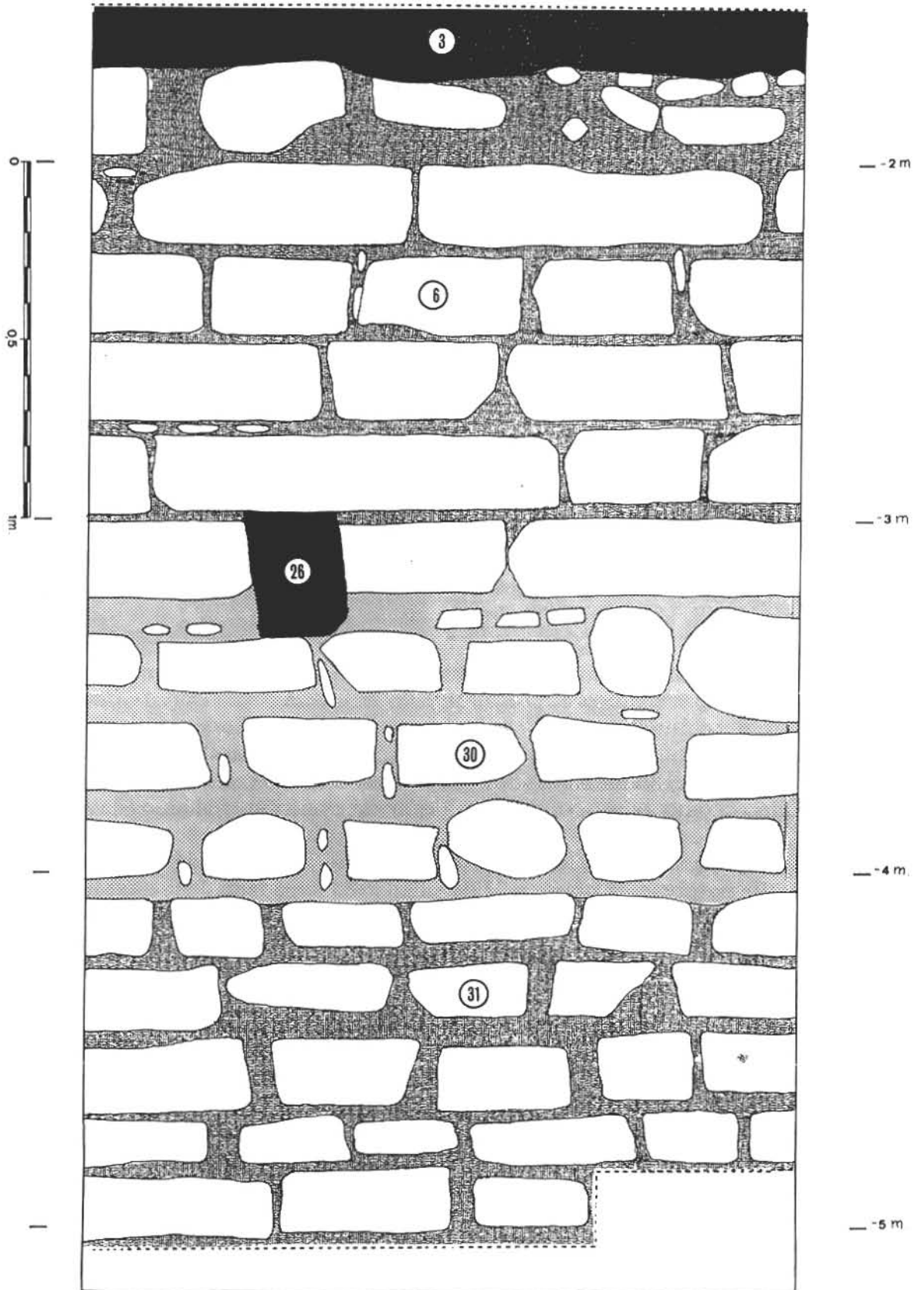
RM · 94 · CORTE 2, PERFIL E ·
