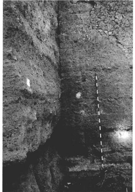
FOTO 8. Técnica de unión de una de las torres al lienzo de muralla, con refuerzo de sillares
