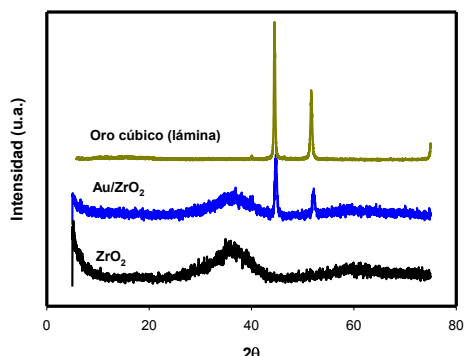
Figura 1.- XRD de ZrO 2 , Au/ZrO 2 y oro puro.
