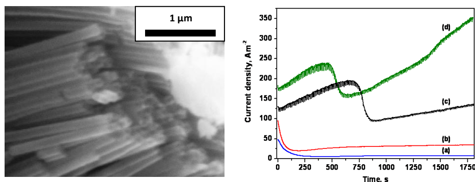
Izquierda: Imagen de SEM de nt-TiO 2 anodizado bajo sonicación a 42V durante 0.5 horas. derecha: Curvas de anodización (J frente al tiempo) de las muestras a) 42 V sin sonicación, b) 60 V sin sonicación, c) 42V bajo sonicación y d) 60V bajo sonicación.
