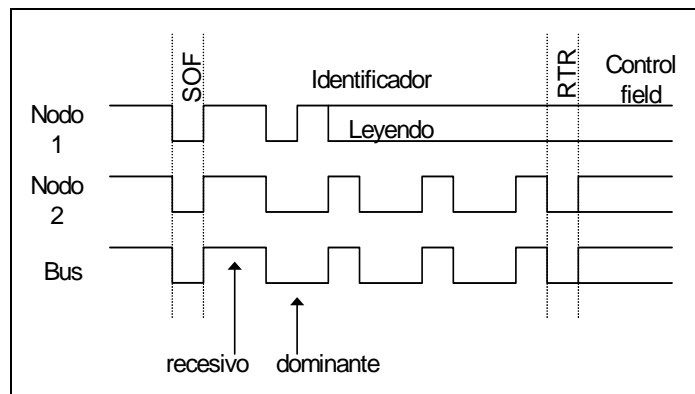
Fig. 2: Arbitración en el bus CAN.
