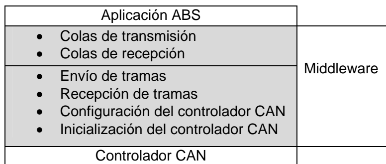
Fig. 7: Estructura de capas de la aplicación objetivo de las prácticas.
