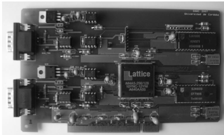
Fig. 3: Fotografía de la placa CAN2PCI.
