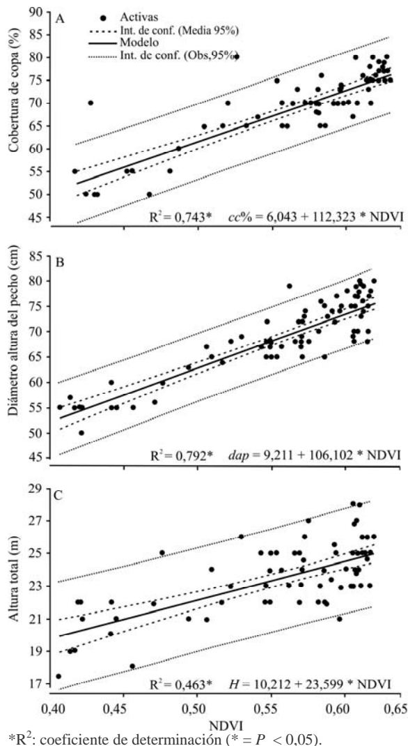
Figura 6. Relación entre el índice de vegetación de diferencia normalizada (NDVI) y tres variables dasométricas de los tipos de bosque de araucaria: a) NDVI y la cobertura de copa (cc, en %), b) NDVI y el diámetro altura del pecho (dap, en cm) y c) NDVI y la altura total de los árboles (H, en m). Para una muestra poblacional de terreno n = 74 parcelas.
