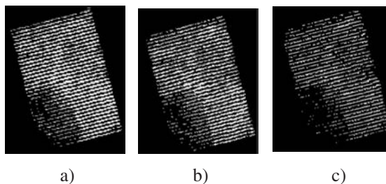
Figura 3. Imágenes de las diferencias de temperatura respecto a los árboles control, obtenidas a partir de las imágenes del AHS para 7:30 a), 9:30 b) y 12:30 c) GMT. En azul: diferencias dentro del intervalo [-2,2 K], en rojo diferencias dentro del intervalo [2,8 K].
