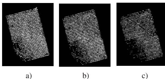
*Figura 4. Imágenes de T_c - T_a obtenidas para 7:30 a), 9:30 b) y las 12:30 GMT c). Los colores para los diferentes intervalos de temperatura son: azul de -2 a 1 K, amarillo de 1 a 4 K y rojo de 4 a 8 K.
