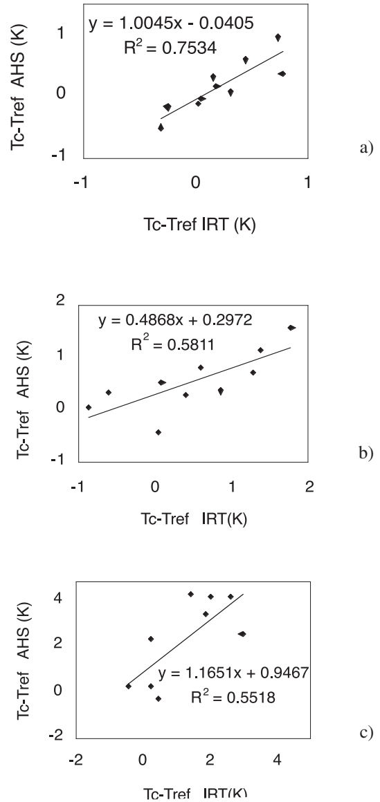
Figura 2. Comparación de las diferencias de temperatura respecto a los puntos de control para cada árbol obtenidas a partir de las imágenes del AHS y medidas con los sensores IRT para las tres horas de vuelo: 7:30 (a), 9:30 (b) y 12:30 GMT (c).
