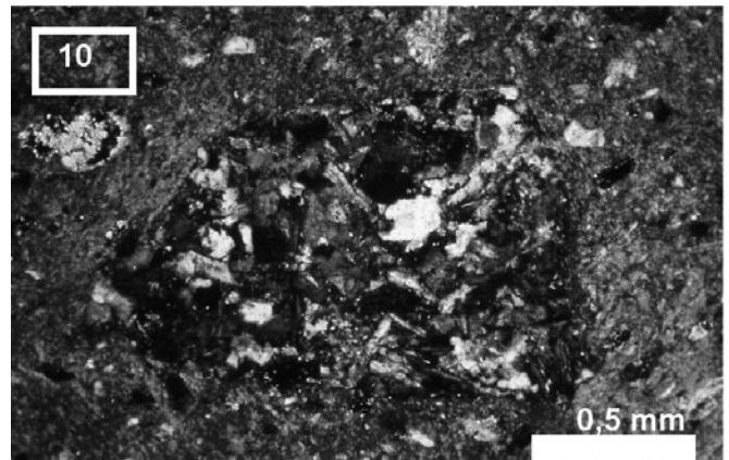
Foto 10: (III). Pasta anisótropa (masépica y eskelsépica) y un clasto volcánico de textura ofítica (micro-gabro ofítico), que contiene plagioclasas (gris y negro) y minerales máficos (píroxenos) parcialmente epidotizados. Polarizadores cruzados.
