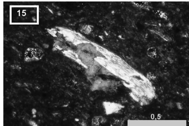
Foto 15: (II). Pasta anisótropa fuertemente roja, clasto de roca metamorfica conteniendo cuarzo-moscovita. Polarizadores cruzados.
