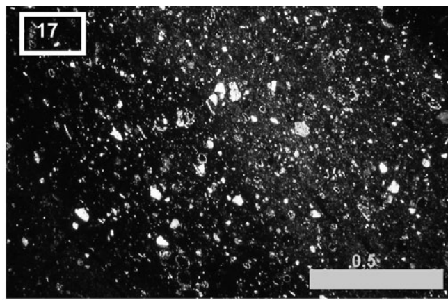
Foto 17: (II). Pasta con diferenciación de núcleo (negro, isótropo) y borde (amarillo oscuro, anisótropo), incluye pequeños clastos minerales (cuarzo, feldespatos). Polarizadores cruzados.
